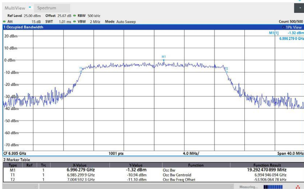
11AX20MIMO-Ant1-6995-PASS
