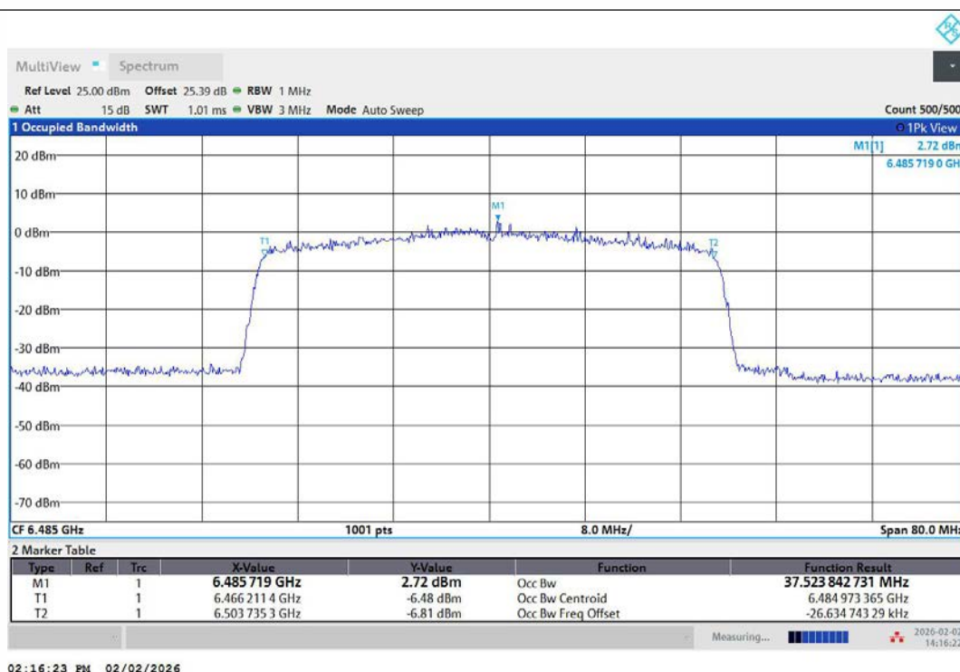
11AX40MIMO-Ant1-6485-PASS
