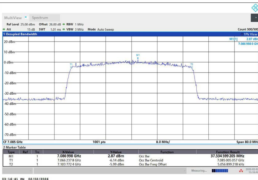
11AX40MIMO-Ant1-7085-PASS
