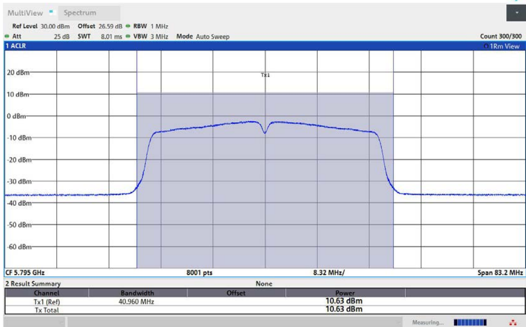
11N40MIMO-Ant1-5795-PASS
