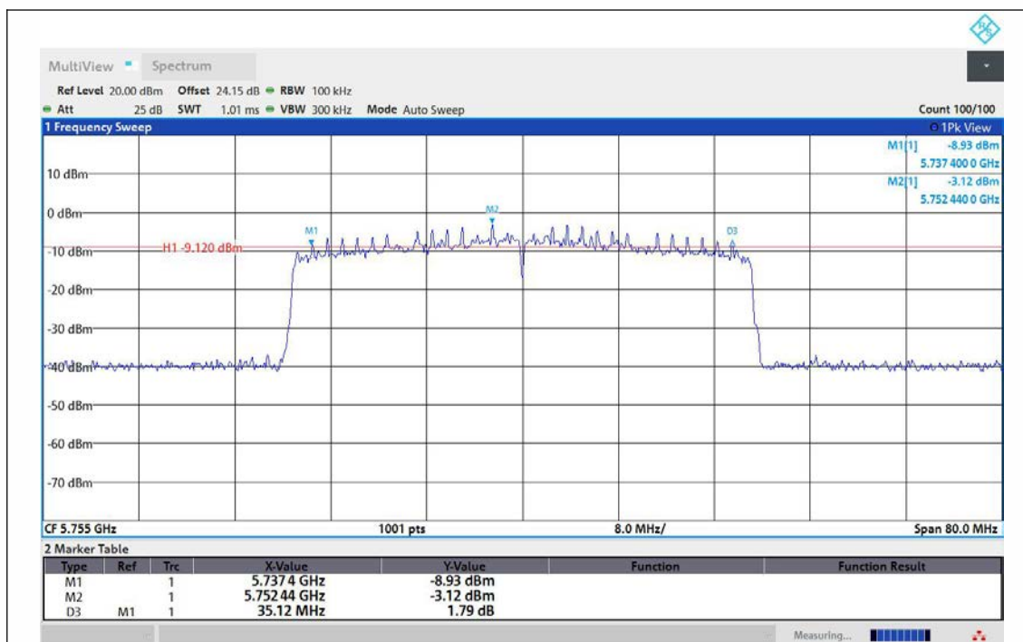
11AX40MIMO-Ant1-5755-PASS
