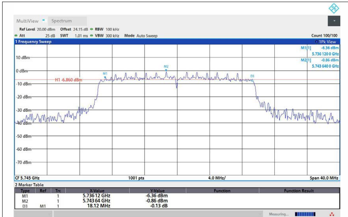
11AX20MIMO-Ant1-5745-PASS
