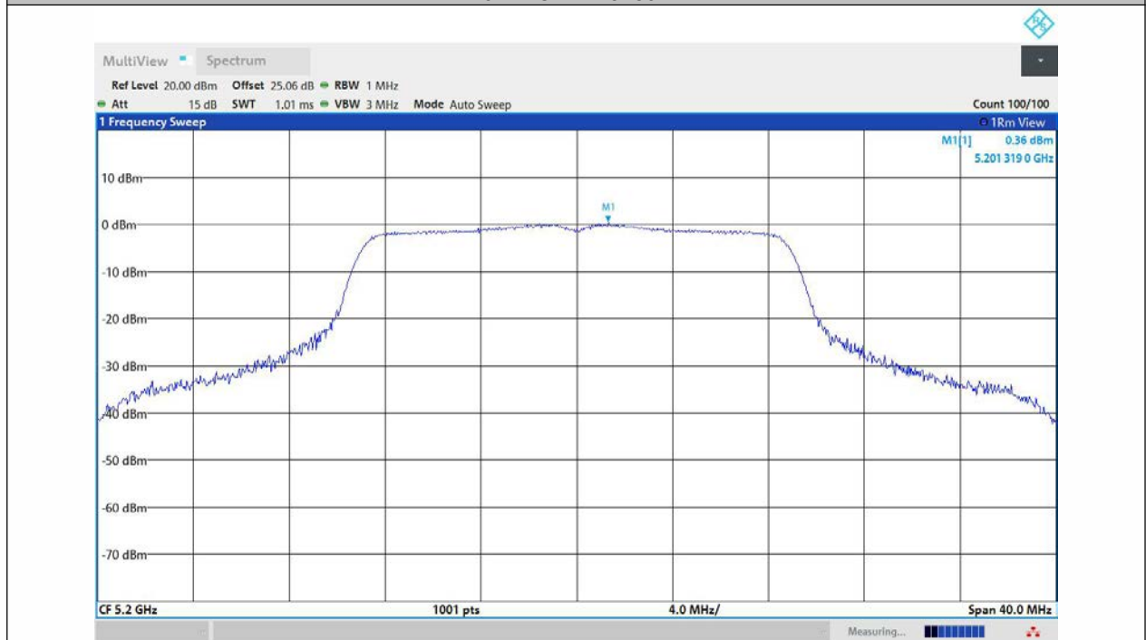
11N20MIMO-Ant1-5200-PASS
