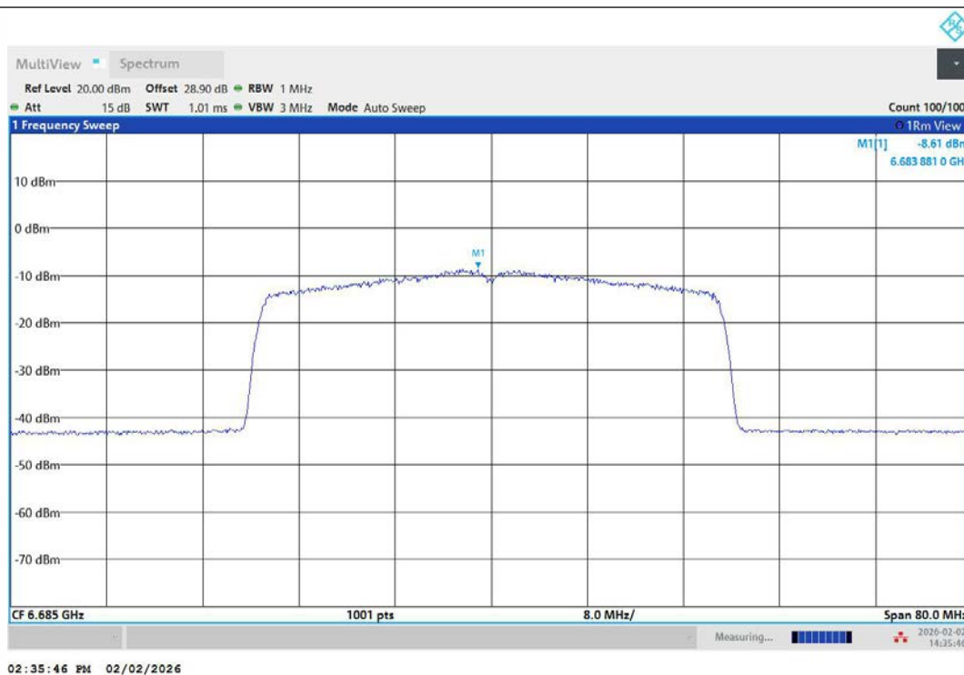
11AX40MIMO-Ant1-6685-PASS
