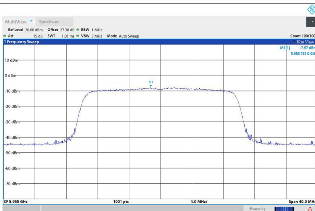
11AX20MIMO-Ant1-5955-PASS
