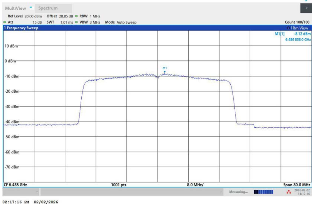
11AX40MIMO-Ant1-6485-PASS
