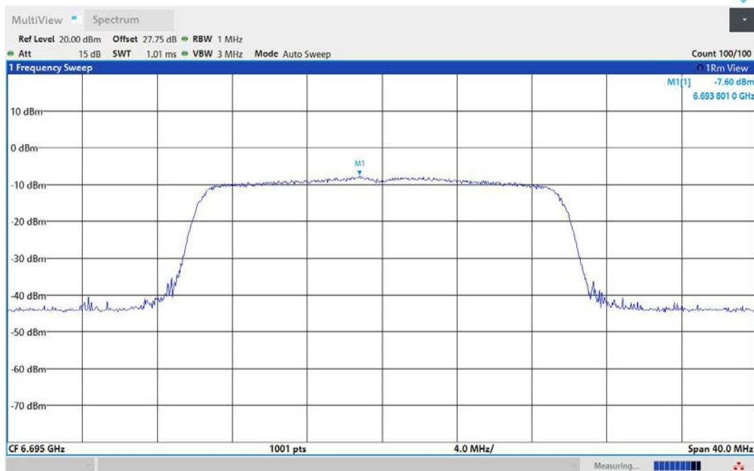
11AX20MIMO-Ant1-6695-PASS
