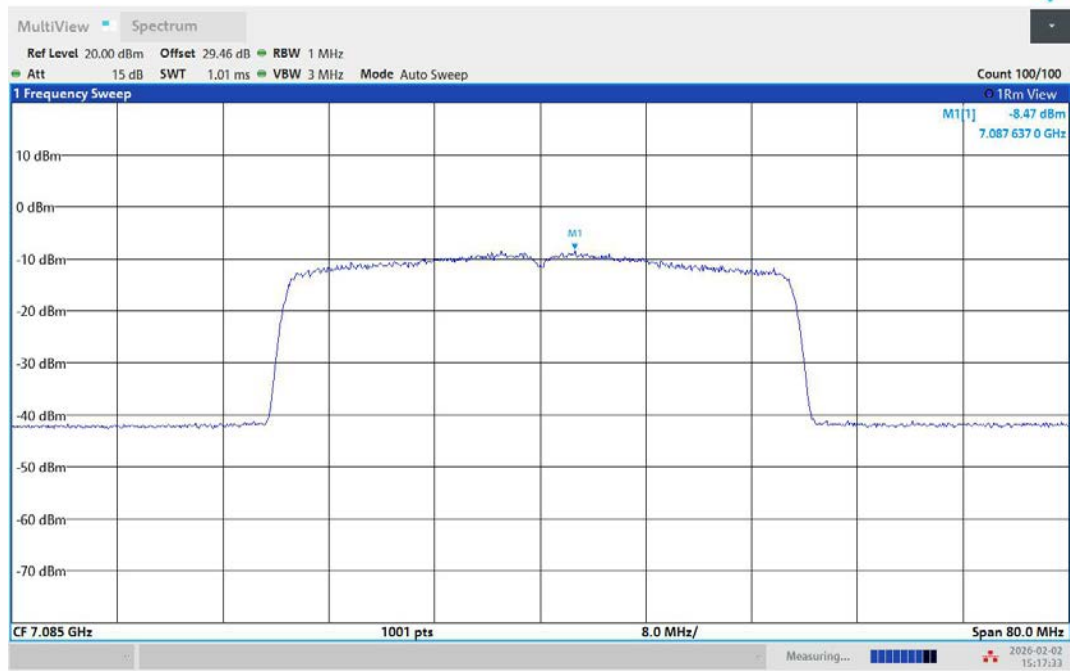
11AX40MIMO-Ant1-7085-PASS
