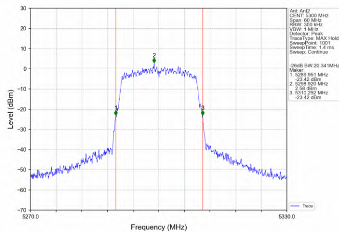
802.11n(HT20)_MCH_5300MHz_Ant2_NTNV
