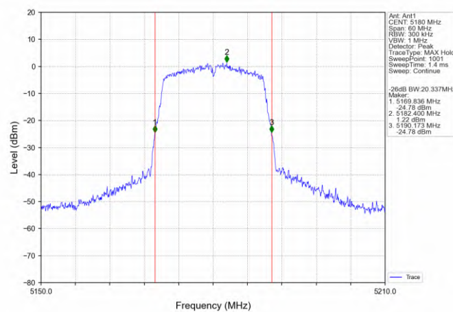
802.11n(HT20)_LCH_5180MHz_Ant1_NTNV
