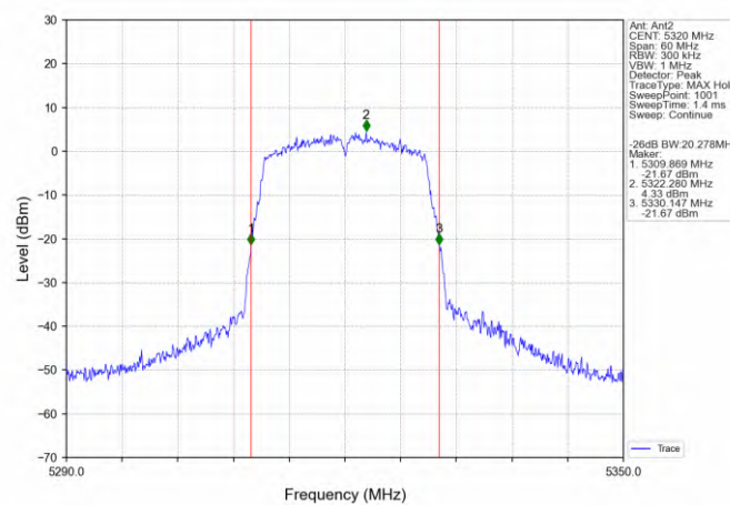
802.11n(HT20)_HCH_5320MHz_Ant2_NTNV
