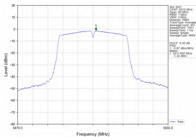
802.11n(HT40)_LCH_5510MHz_Ant1_NTNV
