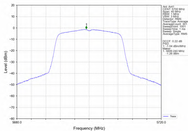
802.11n(HT20)_HCH_5700MHz_Ant1_NTNV
