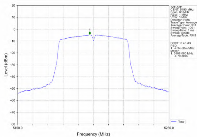
802.11n(HT40)_LCH_5190MHz_Ant1_NTNV
