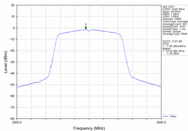
802.11n(HT20)_HCH_5320MHz_Ant1_NTNV
