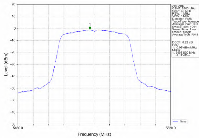
802.11n(HT20)_LCH_5500MHz_MIMO_NTNV
