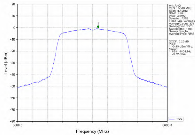
802.11n(HT20)_MCH_5580MHz_MIMO_NTNV
