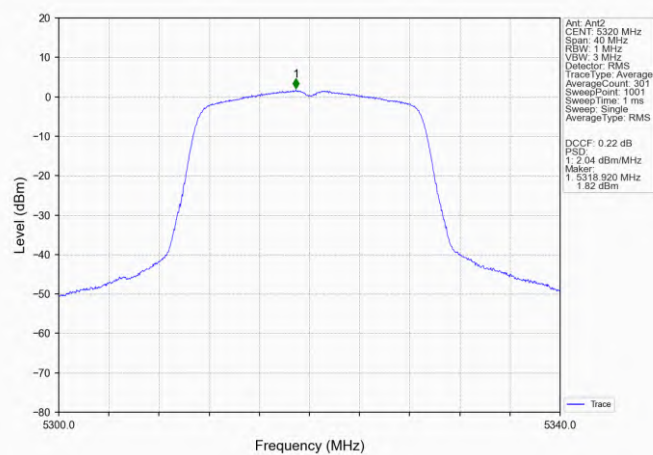
802.11n(HT20)_HCH_5320MHz_Ant2_NTNV
