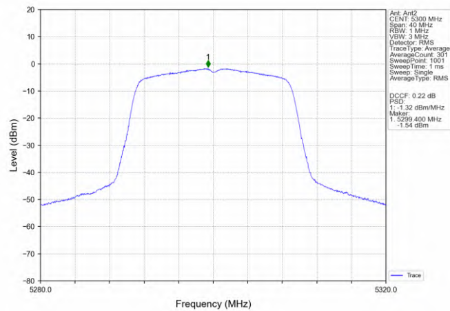
802.11n(HT20)_MCH_5300MHz_MIMO_NTNV
