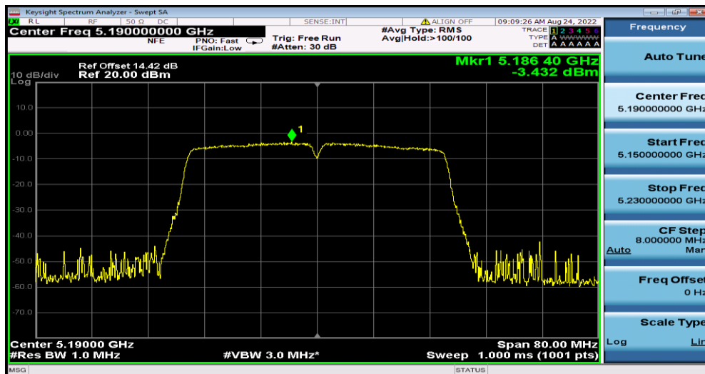
11N40MIMO_Ant1_5190
