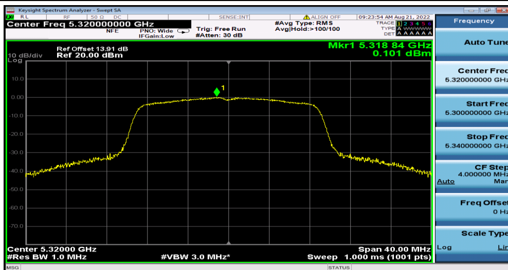
11N20MIMO_Ant1_5320
