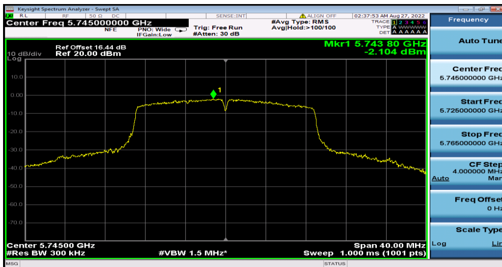
11N20MIMO_Ant2_5745
