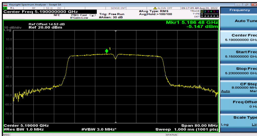
11N40MIMO_Ant2_5190
