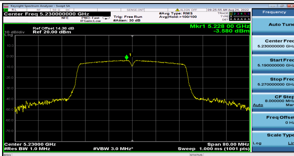
11N40MIMO_Ant1_5230
