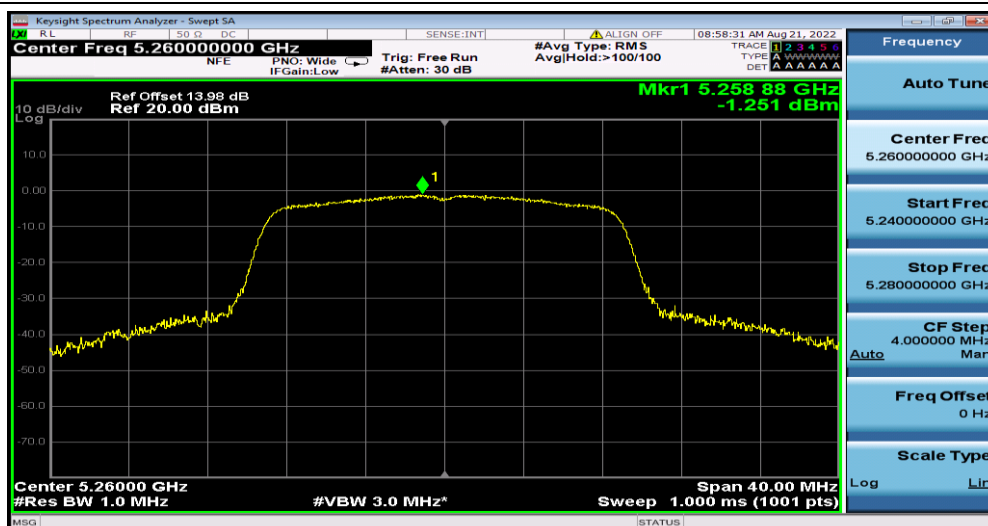
11N20MIMO_Ant1_5260
