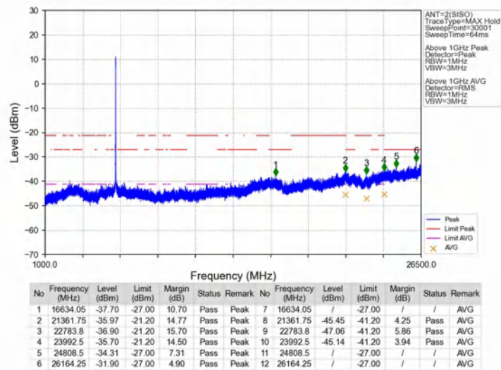
802.11a_MCH_5785MHz_Ant2_NTNV
