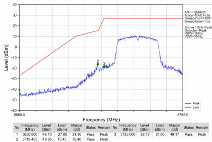
802.11ac(VHT40)_LCH_5755MHz_Ant1_NTNV
