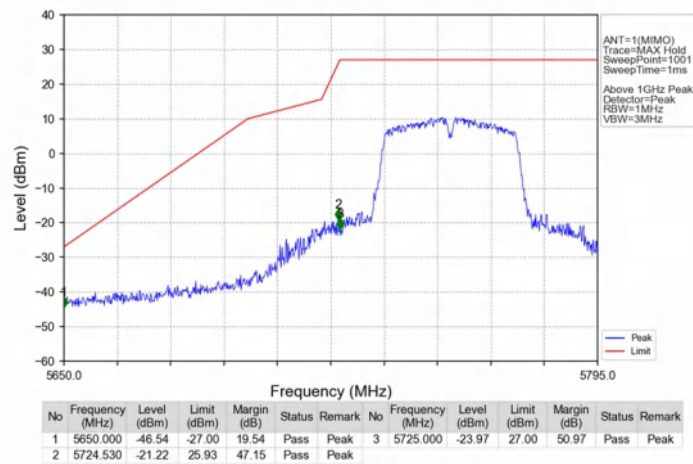
802.11n(HT40)_LCH_5755MHz_Ant1_NTNV
