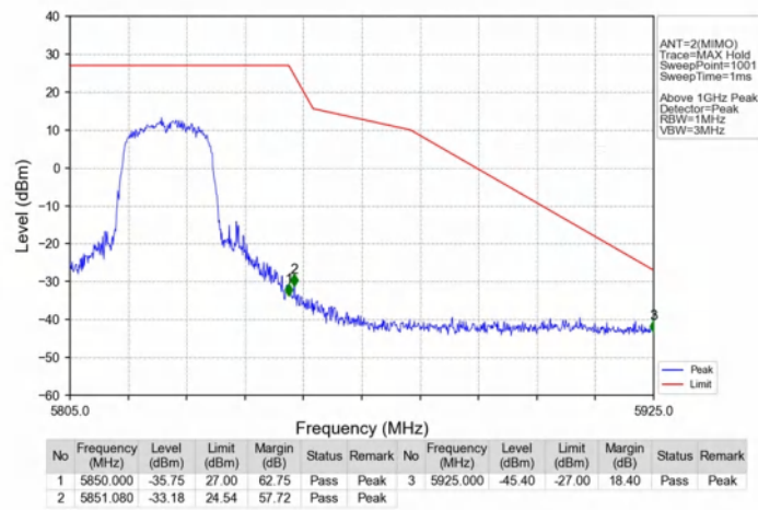
802.11n(HT20)_HCH_5825MHz_Ant2_NTNV
