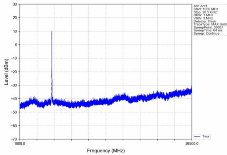
802.11n(HT40)_LCH_5755MHz_Ant1_NTNV
