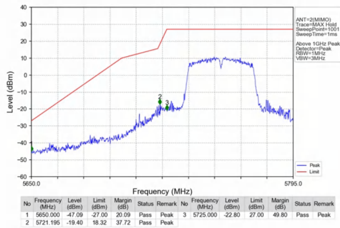
802.11ac(VHT40)_LCH_5755MHz_Ant2_NTNV
