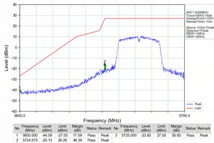
802.11n(HT40)_LCH_5755MHz_Ant2_NTNV
