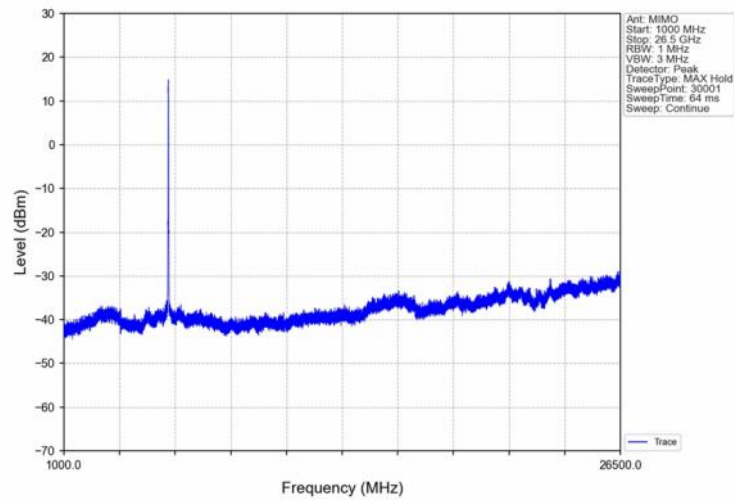
802.11n(HT20)_MCH_5785MHz_MIMO_NTNV
