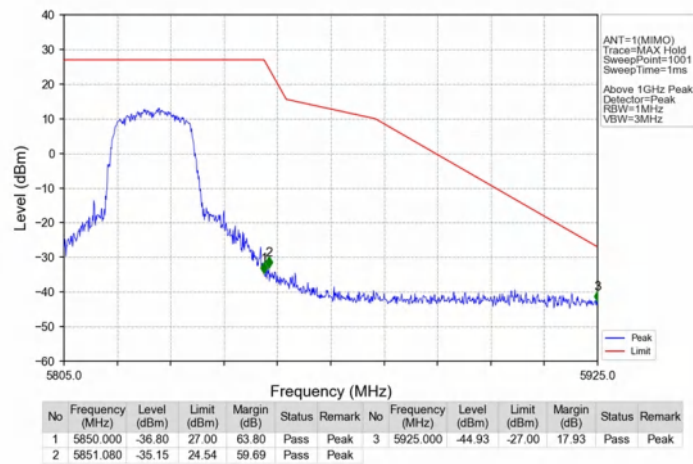
802.11n(HT20)_HCH_5825MHz_Ant1_NTNV
