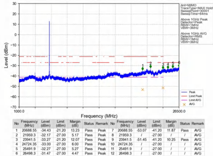
802.11n(HT20)_HCH_5825MHz_MIMO_NTNV
