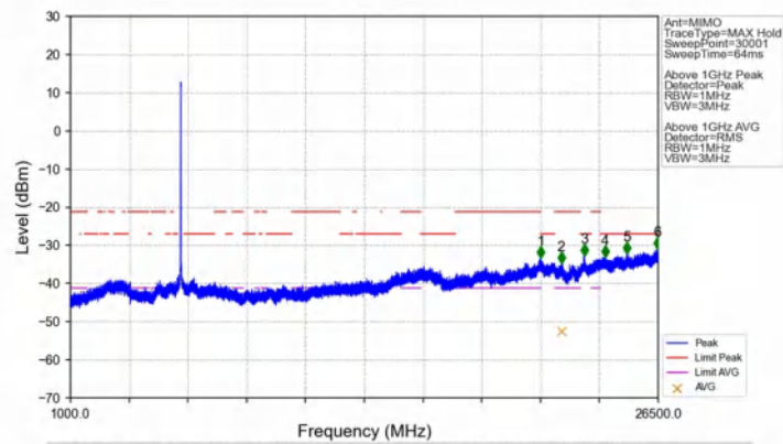
802.11n(HT20)_MCH_5785MHz_MIMO_NTNV
