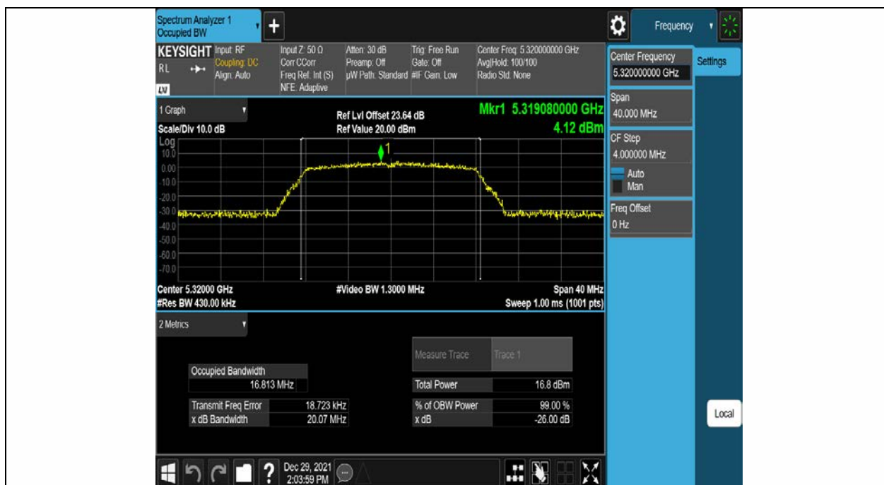
11A Ant1 5320
