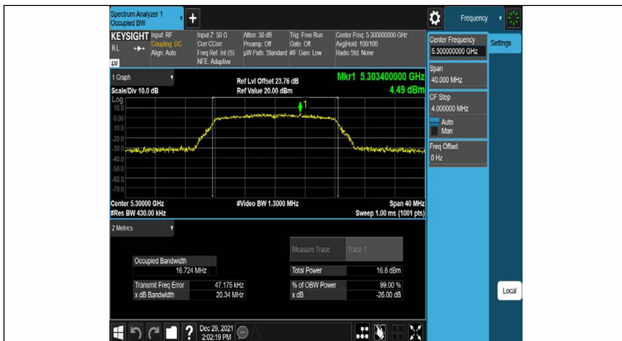
11A Ant1 5300
