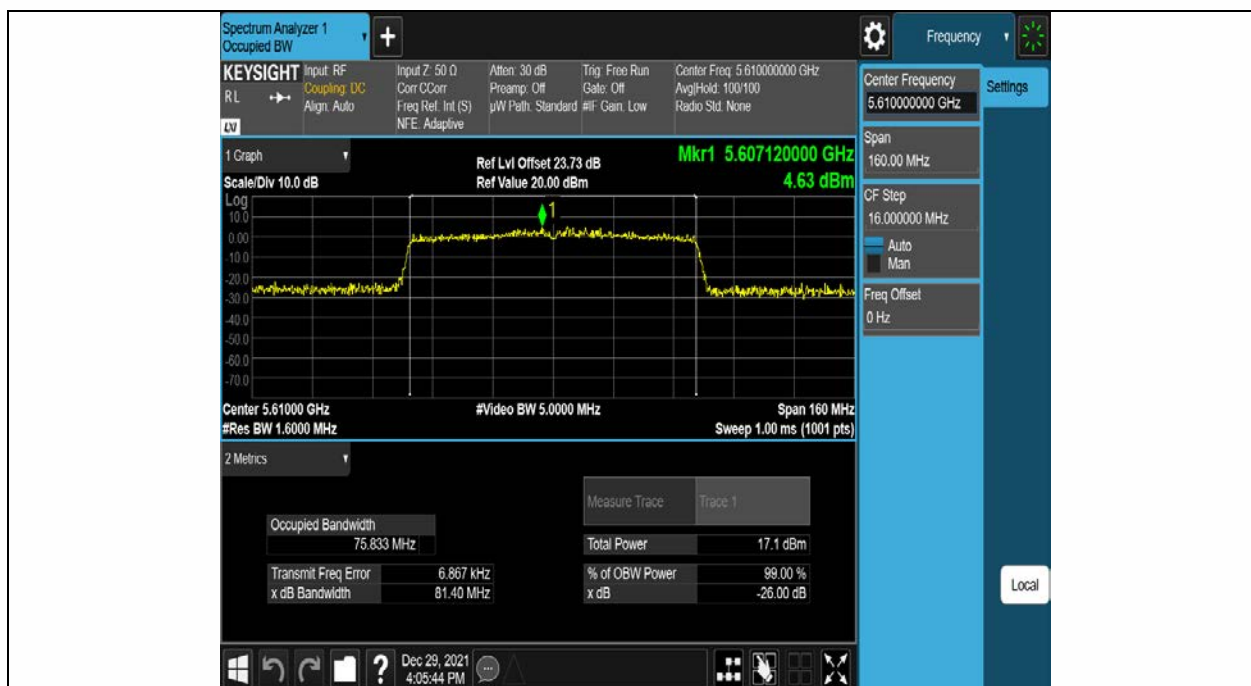
11AC80SISO Ant1 5610
