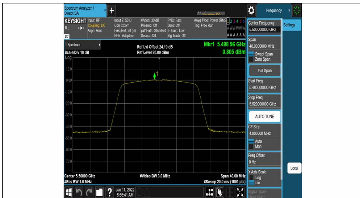
11N20SISO Ant1 5500
