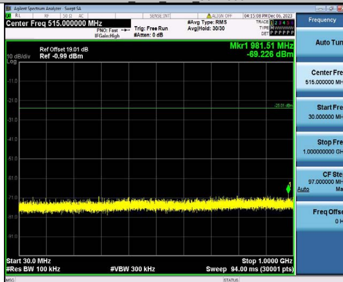
11B_Ant2_2412_30~1000
