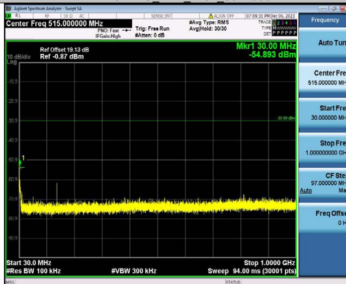
11N40MIMO_Ant2_2437_30~1000
