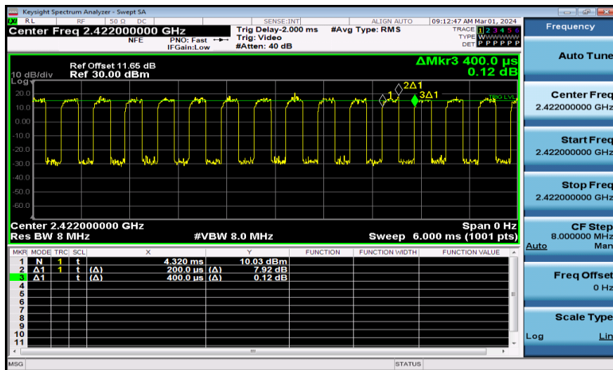
NTNV-11AX40MIMO-Ant1-2422
