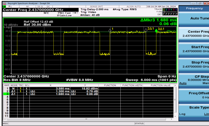
NTNV-11N20MIMO-Ant2-2437
