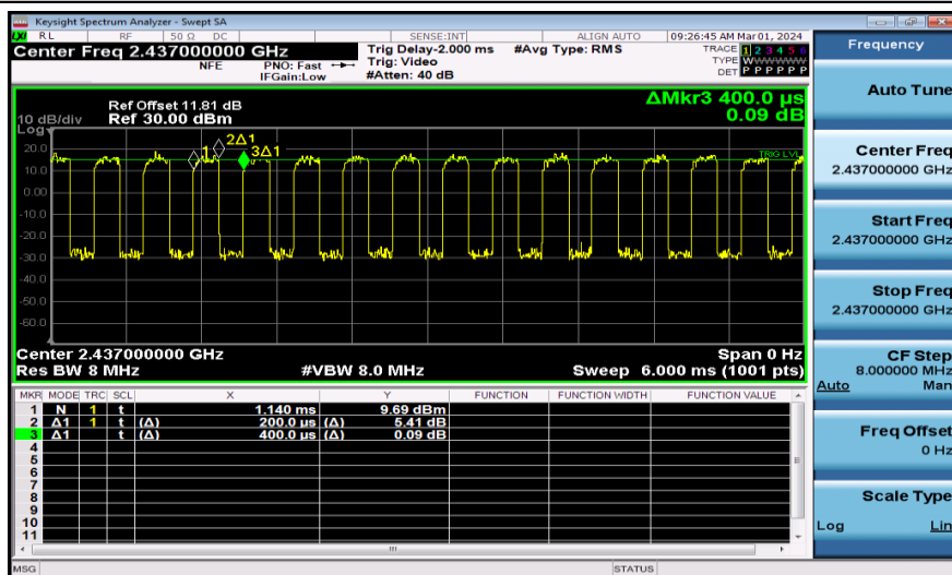
NTNV-11AX40MIMO-Ant1-2437
