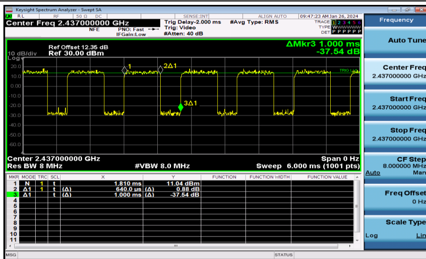
NTNV-11N40MIMO-Ant1-2437
