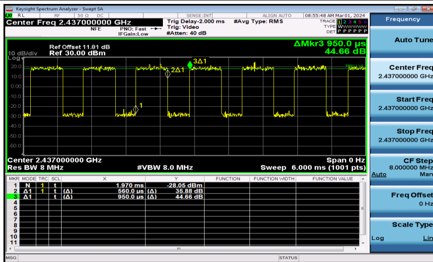
NTNV-11AX20MIMO-Ant1-2437
