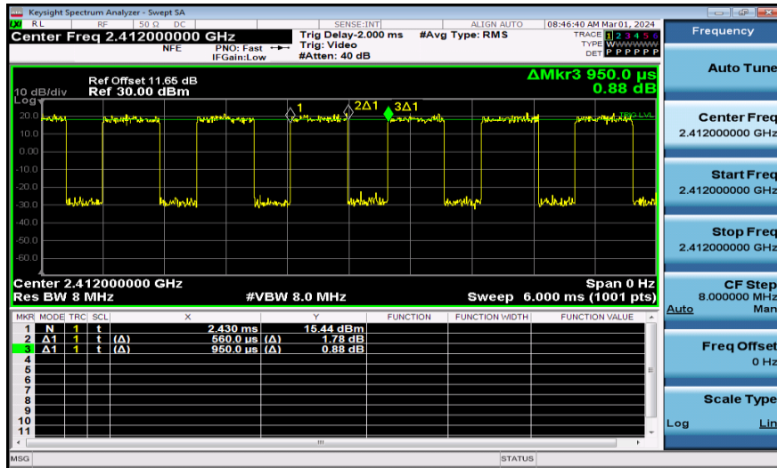
NTNV-11AX20MIMO-Ant1-2412
