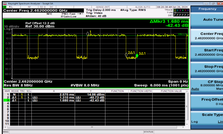
NTNV-11N20MIMO-Ant1-2462
