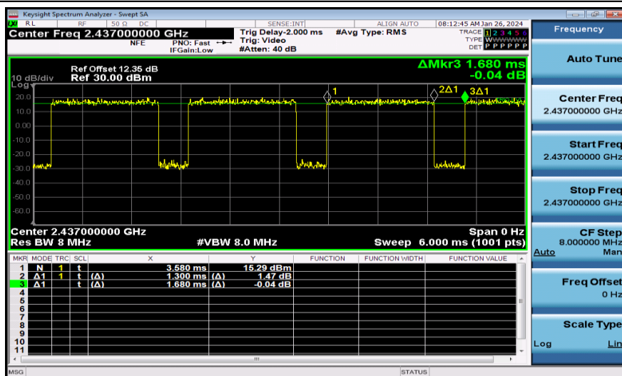
NTNV-11N20MIMO-Ant1-2437
