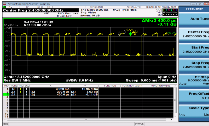
NTNV-11AX40MIMO-Ant1-2452
