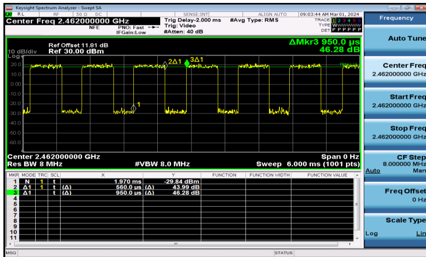
NTNV-11AX20MIMO-Ant1-2462
