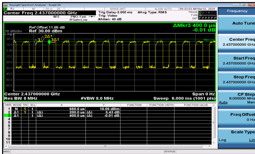
NTNV-11AX40MIMO-Ant2-2437
