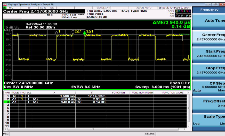
NTNV-11AX20MIMO-Ant2-2437
