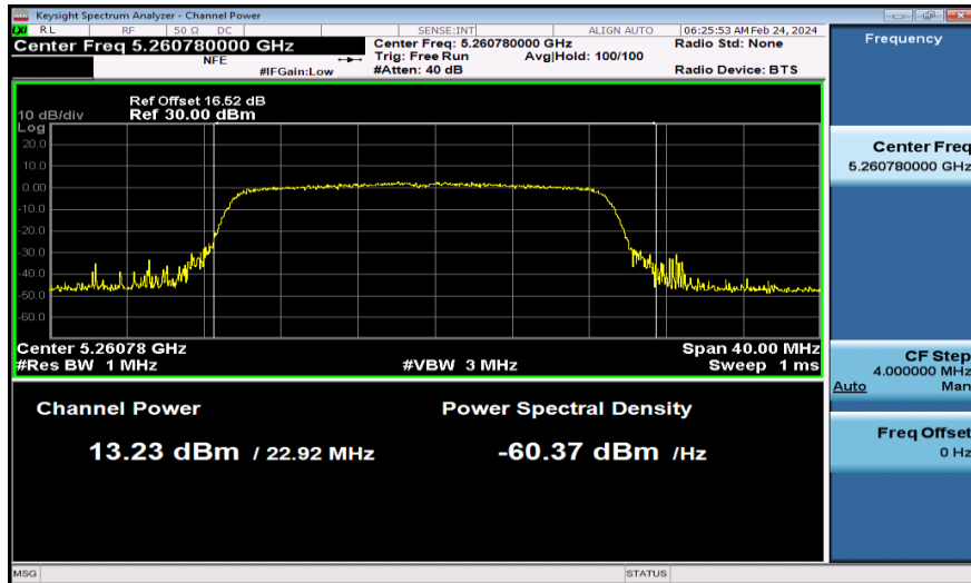
11AX20MIMO-Ant1-5260-PASS
