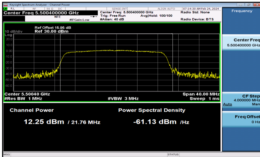
11AX20MIMO-Ant1-5500-PASS
