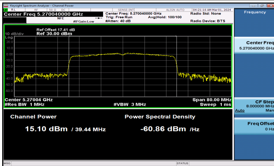
11AX40MIMO-Ant1-5270-PASS
