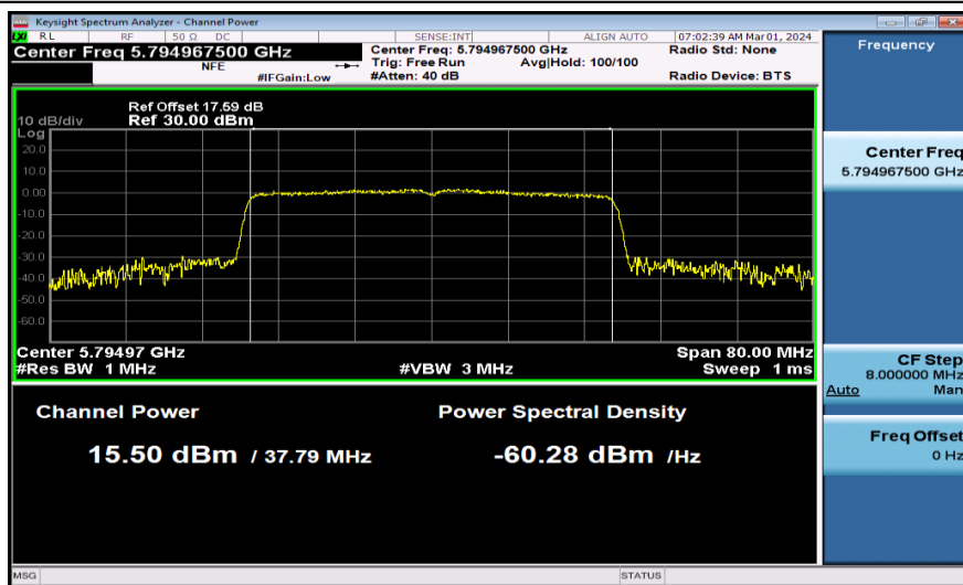
11AX40MIMO-Ant1-5795-PASS
