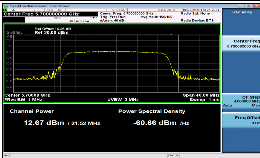
11AX20MIMO-Ant1-5700-PASS
