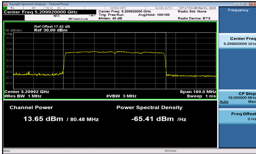
11AX80MIMO-Ant1-5210-PASS
