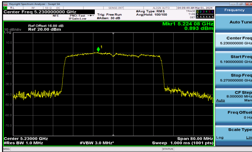
11AX40MIMO-Ant1-5230-PASS
