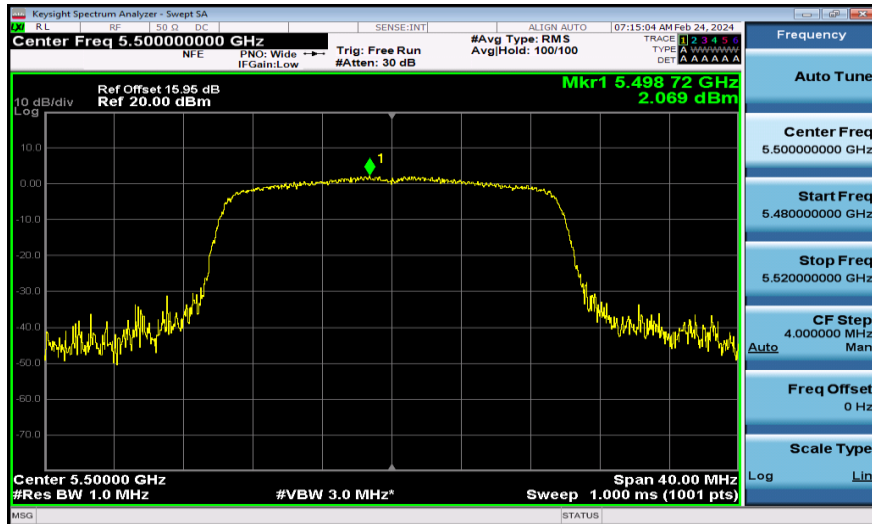
11AX20MIMO-Ant1-5500-PASS
