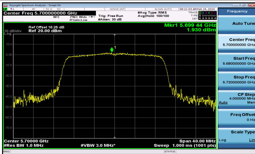
11AX20MIMO-Ant1-5700-PASS
