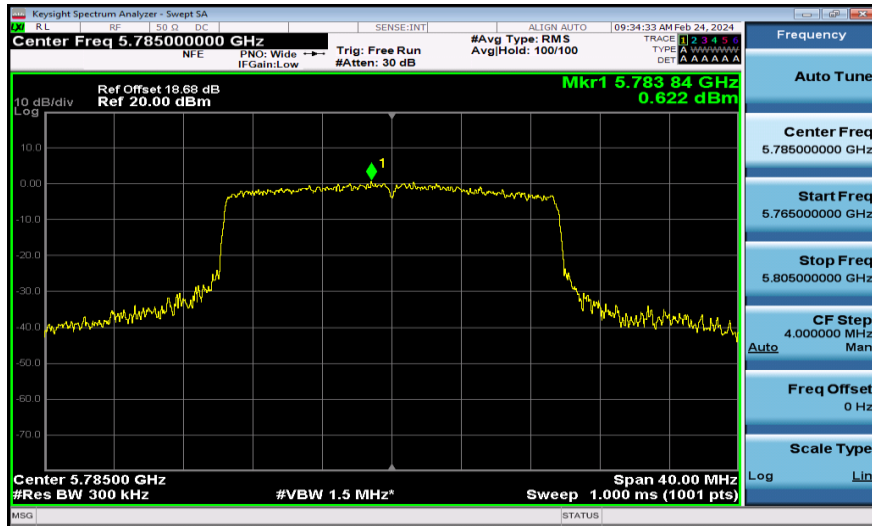
11AX20MIMO-Ant1-5785-PASS
