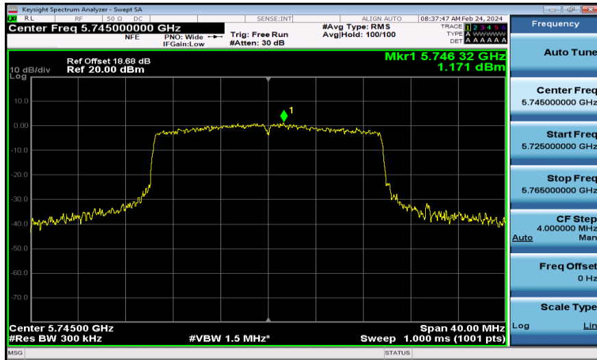
11AX20MIMO-Ant1-5745-PASS
