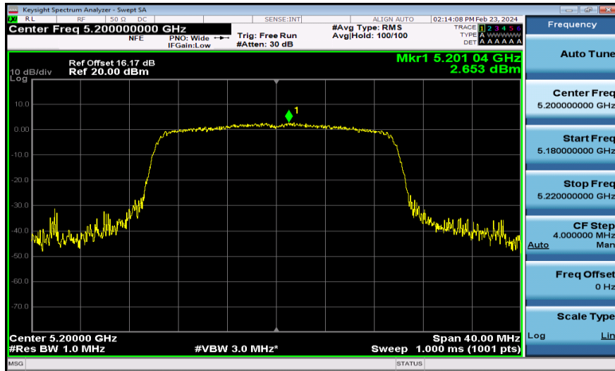
11AX20MIMO-Ant1-5200-PASS
