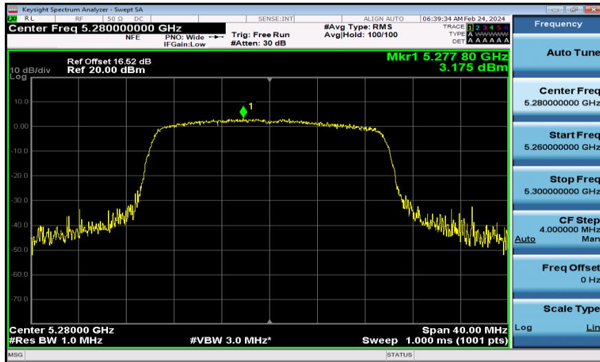
11AX20MIMO-Ant1-5280-PASS
