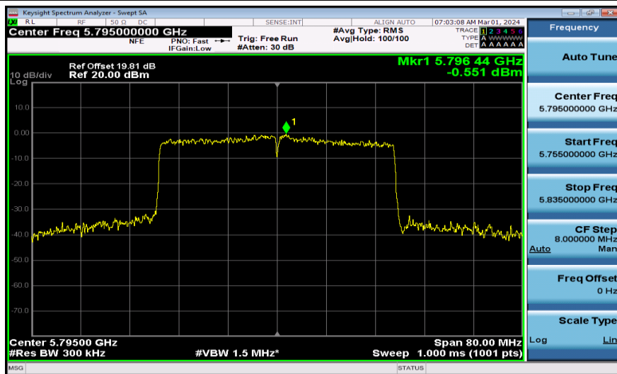
11AX40MIMO-Ant1-5795-PASS
