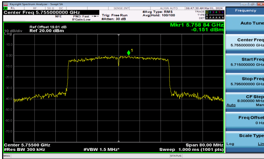
11AX40MIMO-Ant1-5755-PASS
