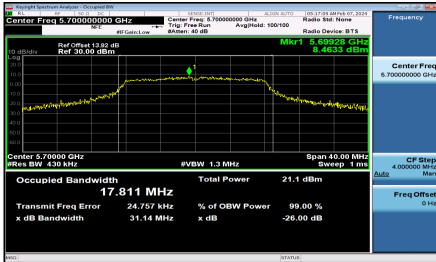
11A-Ant1-5700
