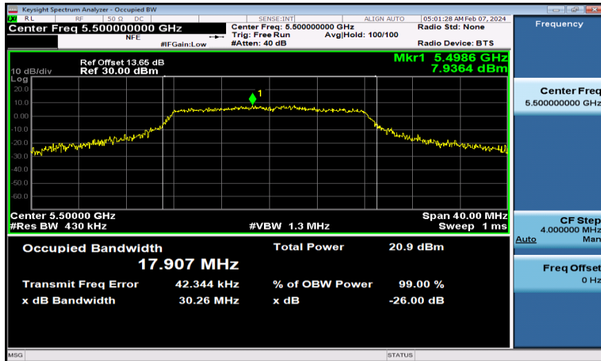
11A-Ant1-5500
