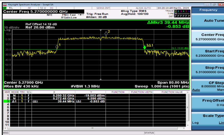
11AX40MIMO-Ant1-5270
