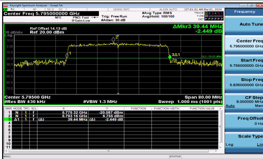
11AX40MIMO-Ant1-5795
