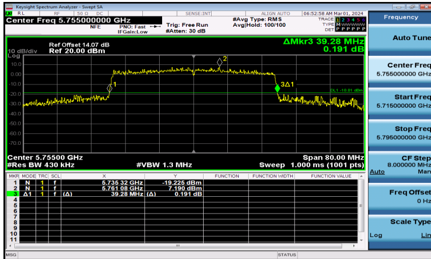
11AX40MIMO-Ant2-5755
