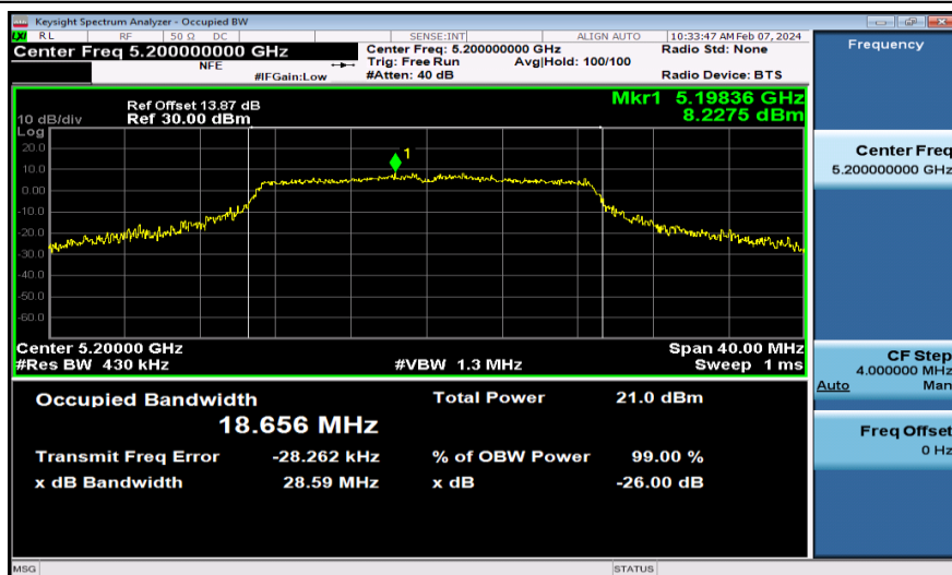
11N20MIMO-Ant1-5200
