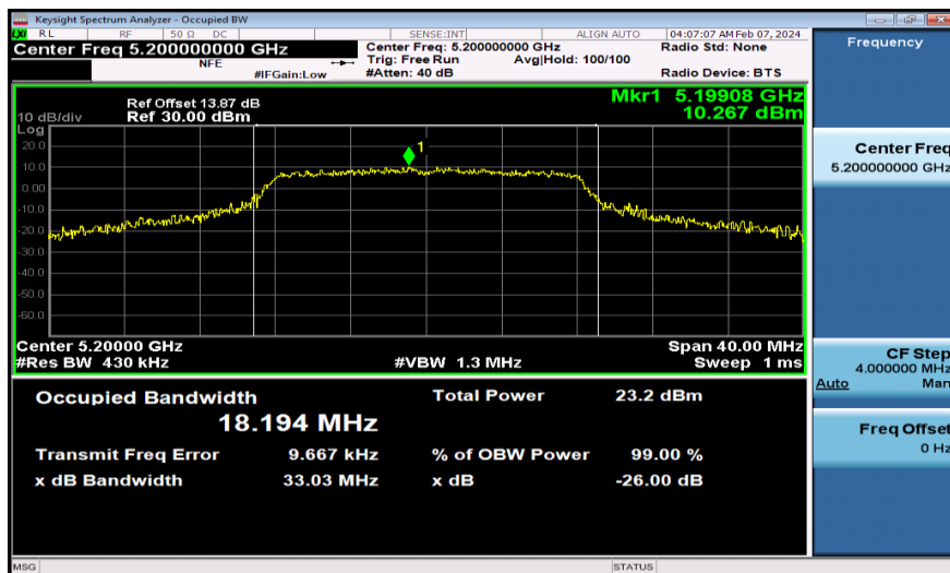
11A-Ant1-5200
