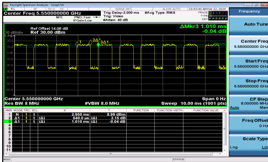
NTNV-11N40MIMO-Ant1-5550
