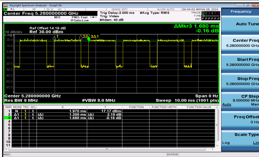
NTNV-11N20MIMO-Ant1-5280
