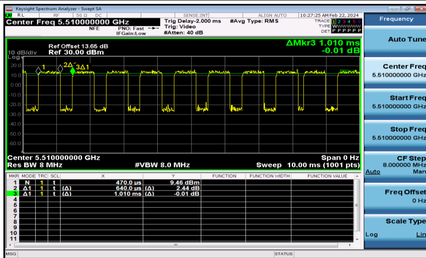
NTNV-11N40MIMO-Ant1-5510
