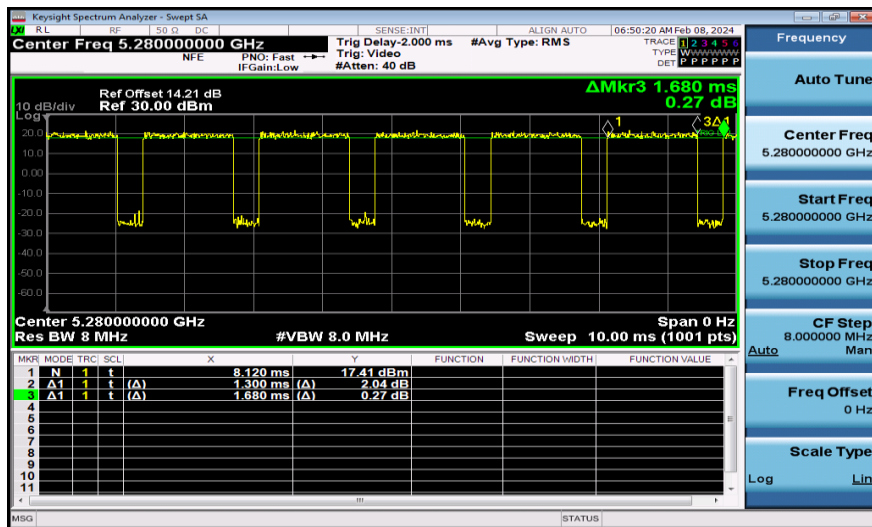
NTNV-11N20MIMO-Ant2-5280
