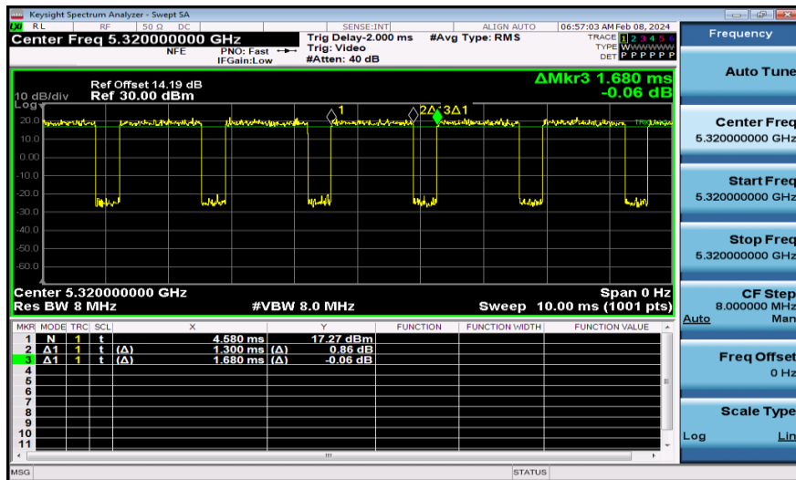
NTNV-11N20MIMO-Ant1-5320
