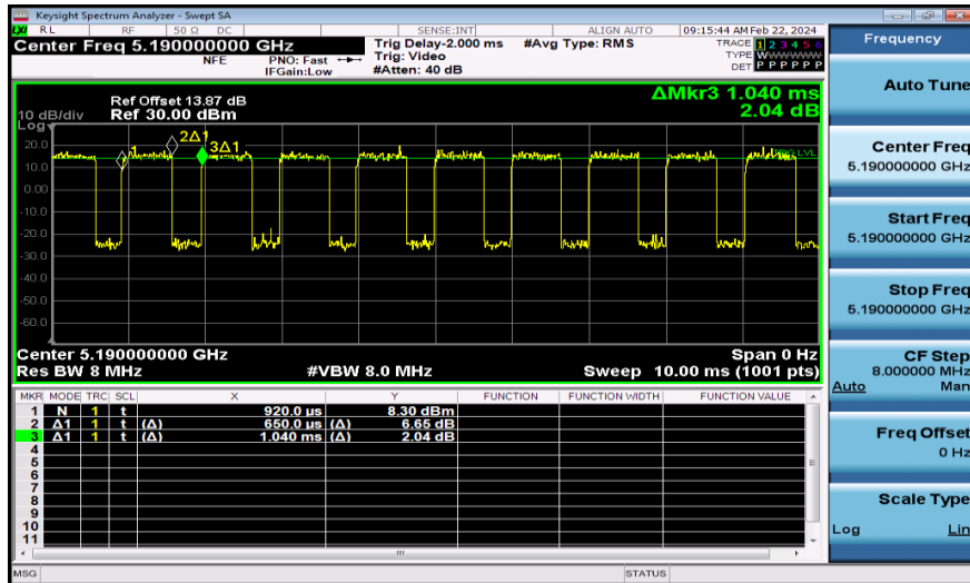
NTNV-11N40MIMO-Ant1-5190
