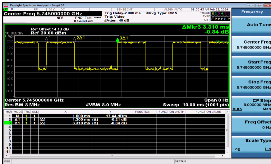
NTNV-11N20MIMO-Ant1-5745
