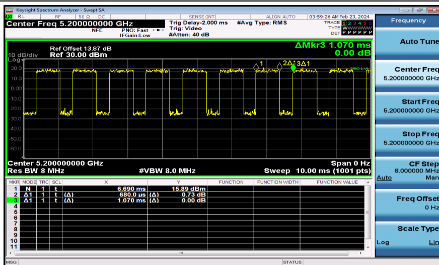
NTNV-11AC20MIMO-Ant1-5200
