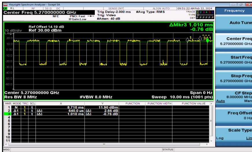
NTNV-11N40MIMO-Ant1-5270
