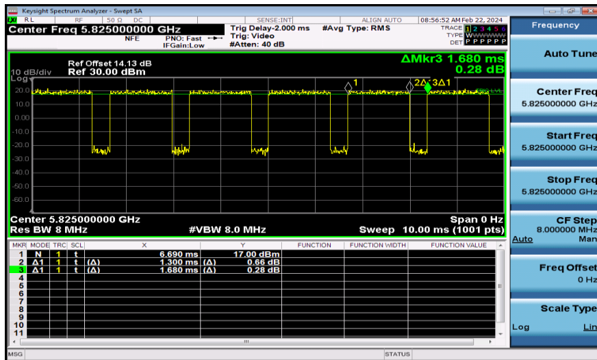
NTNV-11N20MIMO-Ant1-5825
