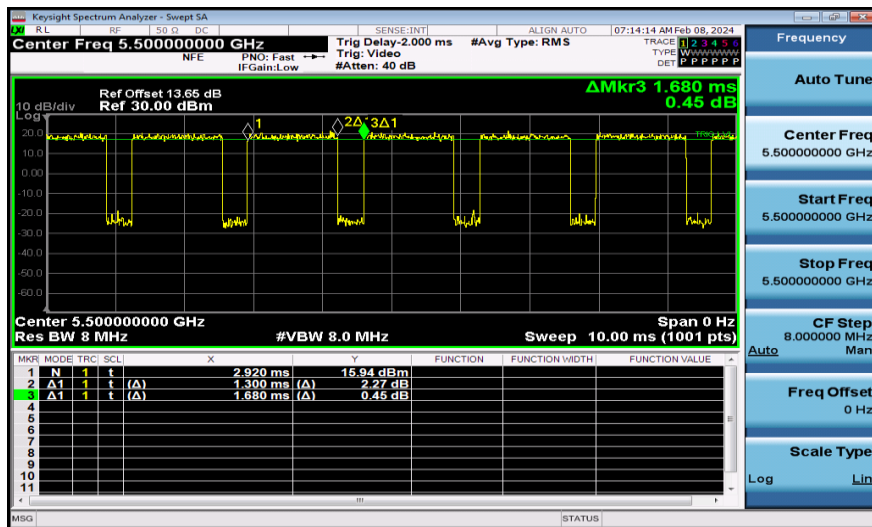
NTNV-11N20MIMO-Ant1-5500
