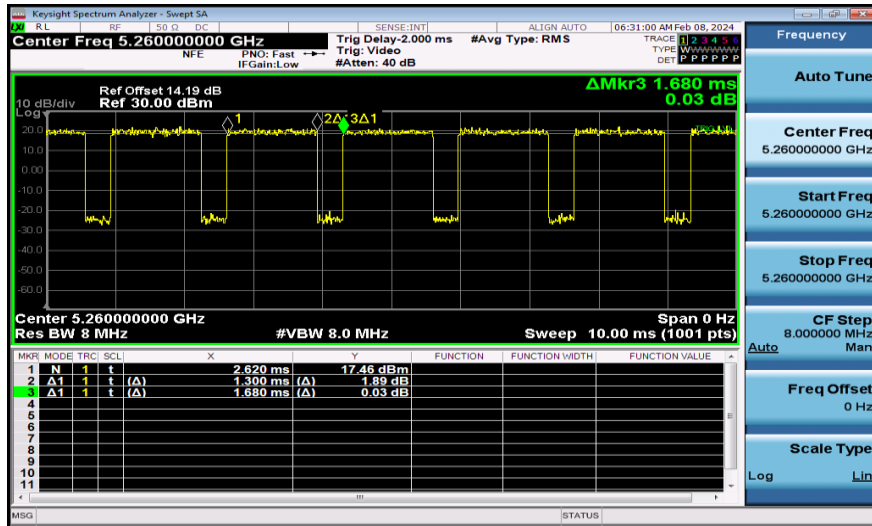
NTNV-11N20MIMO-Ant1-5260
