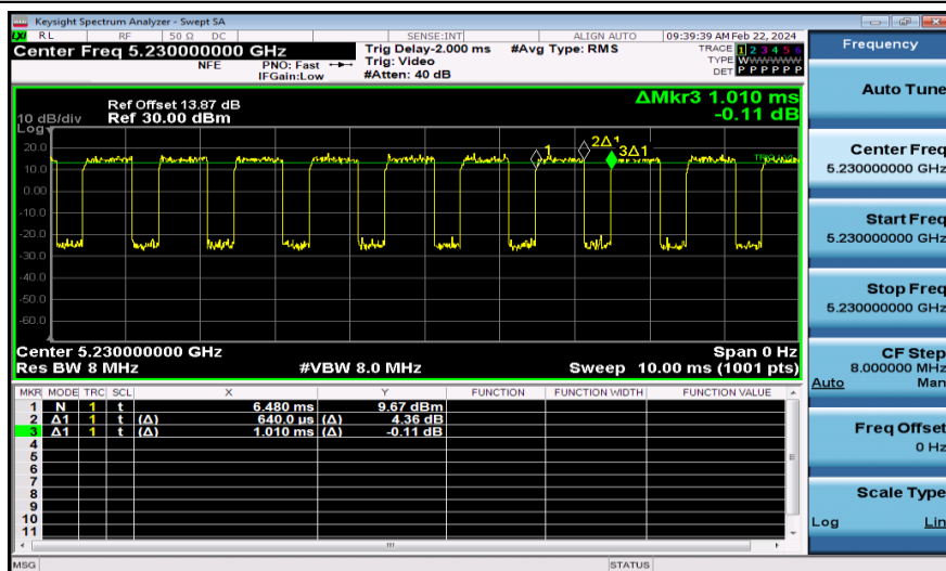
NTNV-11N40MIMO-Ant1-5230
