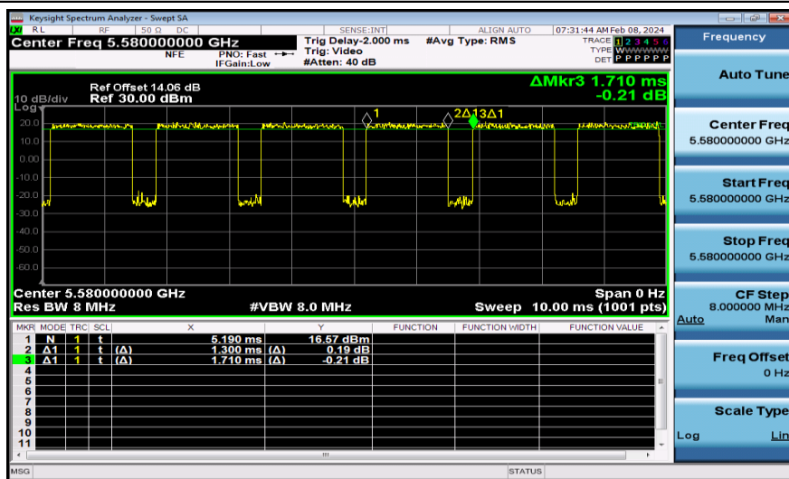
NTNV-11N20MIMO-Ant1-5580
