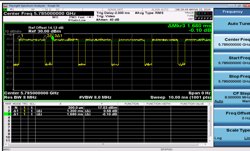
NTNV-11N20MIMO-Ant1-5785
