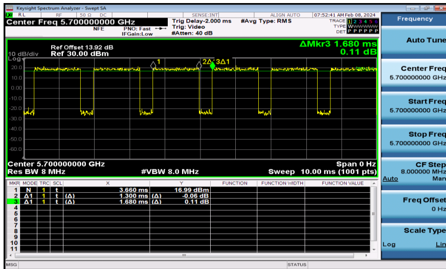
NTNV-11N20MIMO-Ant1-5700
