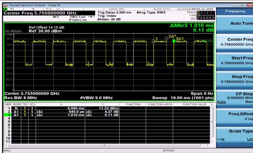
NTNV-11N40MIMO-Ant1-5755
