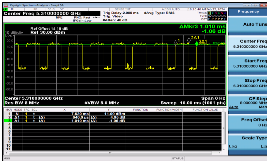
NTNV-11N40MIMO-Ant1-5310
