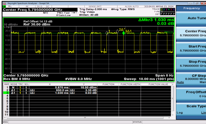
NTNV-11N40MIMO-Ant1-5795
