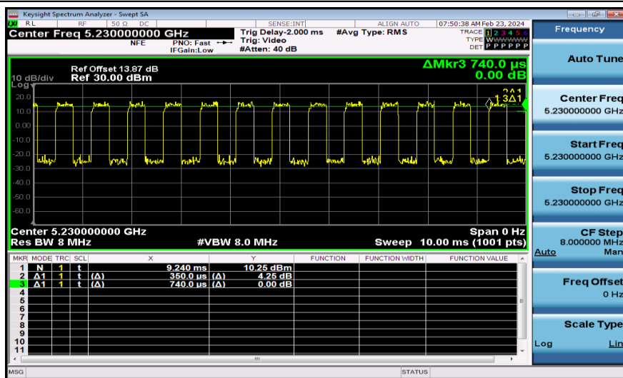
NTNV-11AC40MIMO-Ant1-5230
