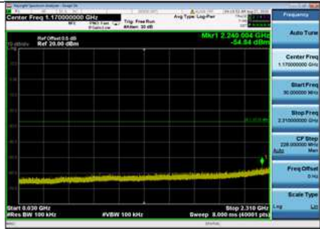
802.11n(HT20),2437MHz,Ant1,Plot 3,30MHz~2310MHz
