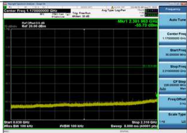
802.11b,2437MHz,Ant1,Plot 3,30MHz~2310MHz
