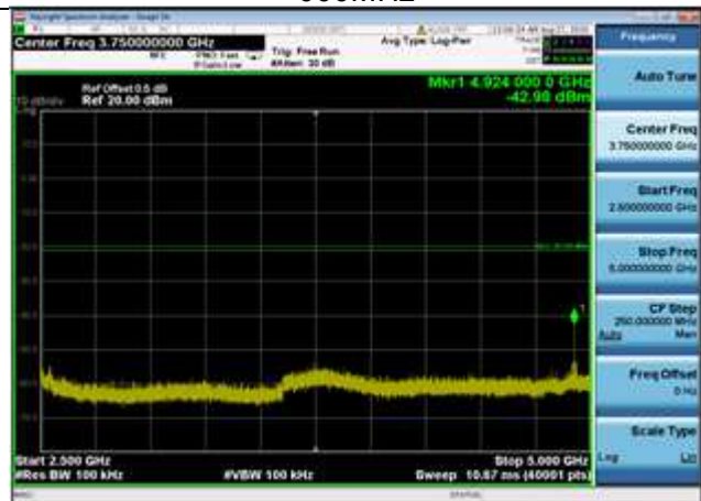
802.11b,2462MHz,Ant0,Plot 4,2500MHz~5000MHz
