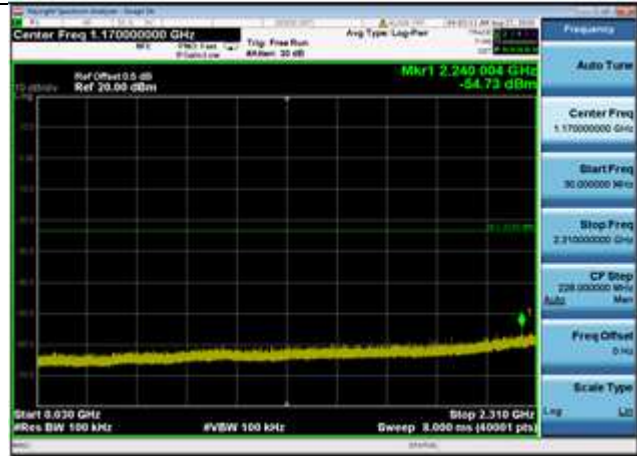
802.11g,2437MHz,Ant1,Plot 3,30MHz~2310MHz
