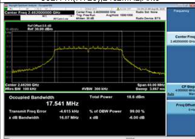
802.11n(HT20),2462MHz,Ant0
