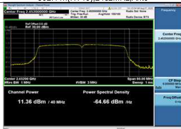
802.11n(HT40),2452MHz,Ant0
