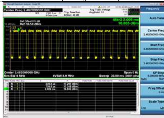
802.11n(HT20),2462MHz,Ant0
