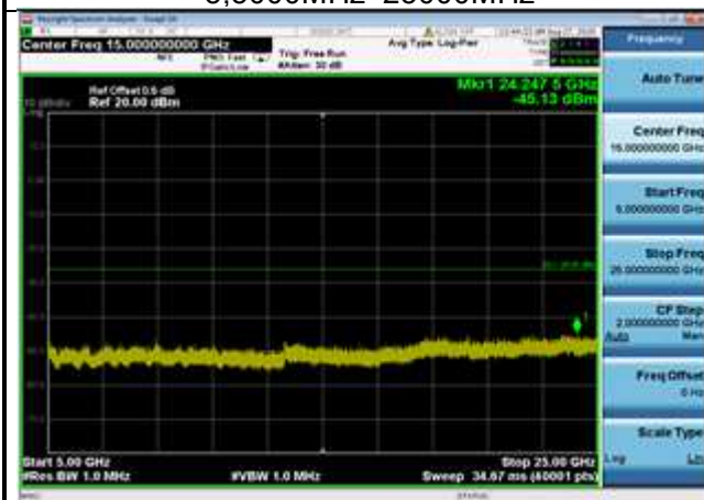
802.11n(HT20),2412MHz,Ant0,Plot 5,5000MHz~25000MHz
