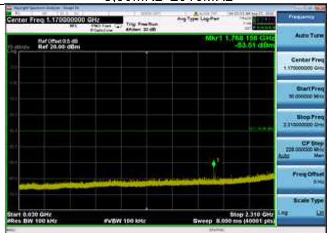
802.11n(HT40),2437MHz,Ant1,Plot 3,30MHz~2310MHz
