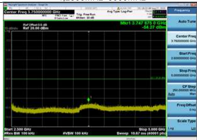
802.11n(HT40),2452MHz,Ant0,Plot 4,2500MHz~5000MHz
