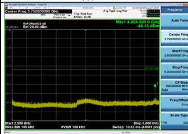
802.11b,2462MHz,Ant1,Plot 4,2500MHz~5 000MHz
