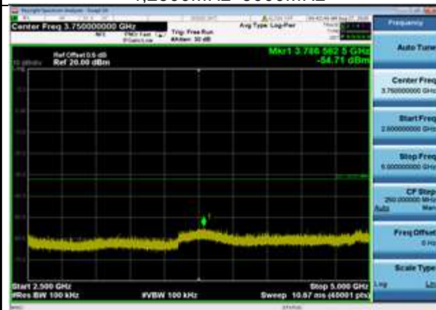
802.11n(HT40),2452MHz,Ant1,Plot 4,2500MHz~5000MHz
