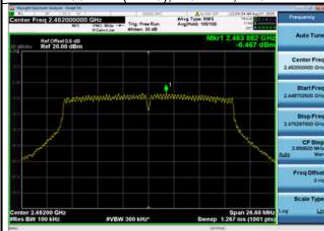
802.11n(HT20),2462MHz,Ant0
