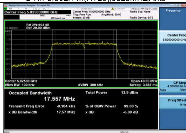
U-NII-3,802.11n(HT20),5825MHz,Ant0
