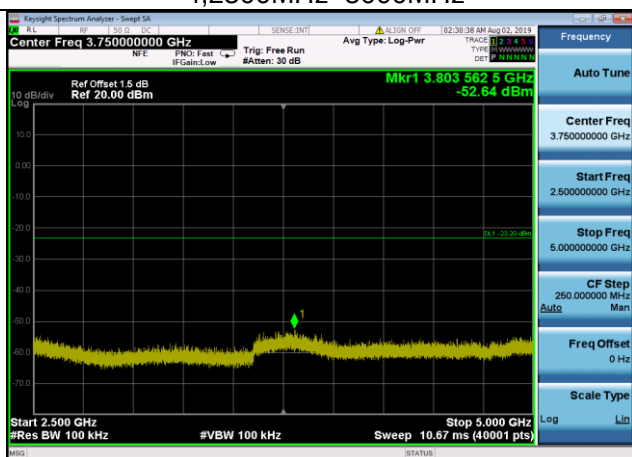
802.11n(HT40),2437MHz,Ant0,Plot 4,2500MHz~5000MHz
