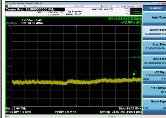
802.11n(HT20),2412MHz,Ant0,Plot 5,5000MHz~25000MHz
