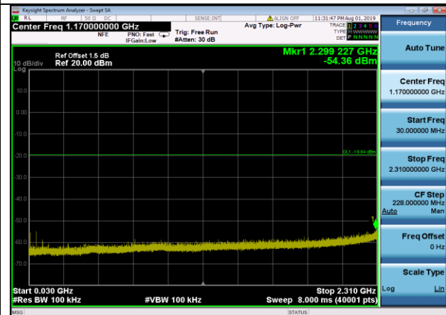
802.11g,2412MHz,Ant0,Plot 3,30MHz~2310MHz
