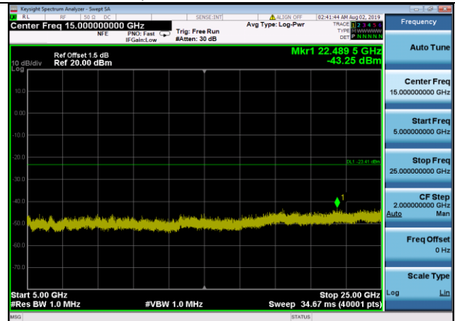
802.11n(HT40),2452MHz,Ant0,Plot 5,5000MHz~25000MHz
