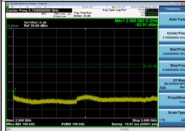
802.11n(HT40),2452MHz,Ant0,Plot 4,2500MHz~5000MHz
