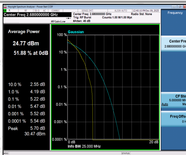
Band41-20MHz-QPSK-41490-1RB#0
