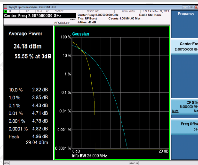
Band41-5MHz-QPSK-41565-1RB#0
