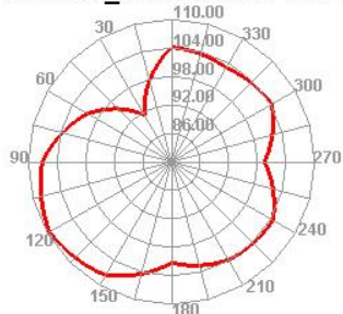
WCDMA_VIII 3088 TIS Phi=45
