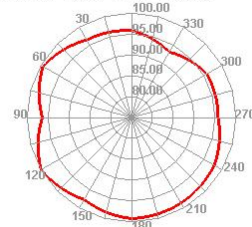
LTE3 1900 TIS Phi=45
