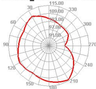
WCDMA_I 10838 TIS Phi=45
