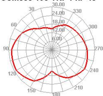
GSM850 190 TRP Phi=45
