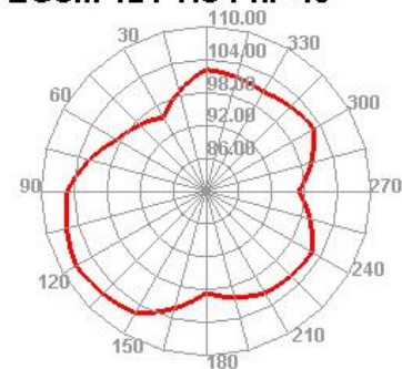
EGSM 124 TIS Phi=45
