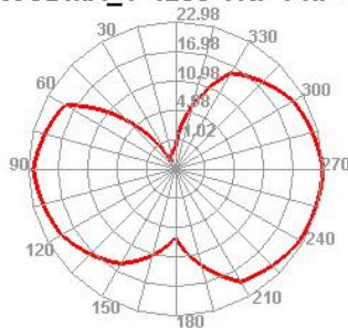
WCDMA_V 4233 TRP Phi=45
