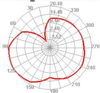
WCDMA_VIII 2788 TRP Phi=45
