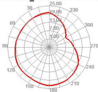
WCDMA_I 9888 TRP Phi=45
