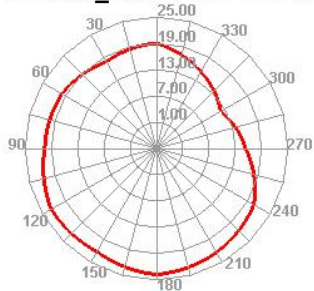
WCDMA_I 9612 TRP Phi=45
