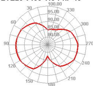
LTE20 6400 TIS Phi=45
