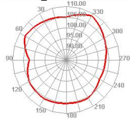
WCDMA_II 9938 TIS Phi=45
