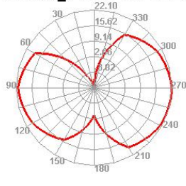
WCDMA_V 4185 TRP Phi=45
