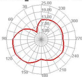
WCDMA_VIII 2863 TRP Phi=45
