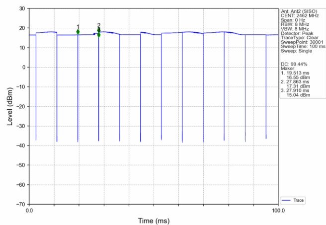
802.11b_HCH_2462MHz_Ant2 (SISO)_NTNV
