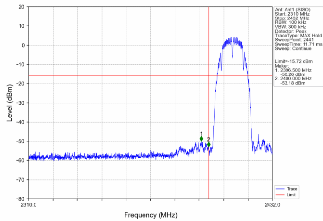
802.11b_LCH_2412MHz_Ant1 (SISO)_NTNV
