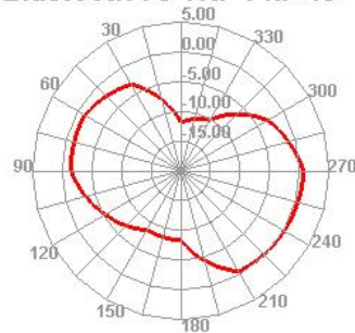
Bluetooth 78 TRP Phi=45
