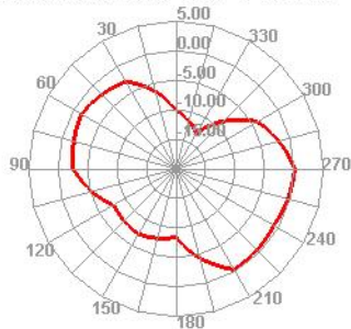
Bluetooth 39 TRP Phi=45
