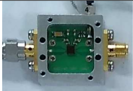
5-18GHz MPA
