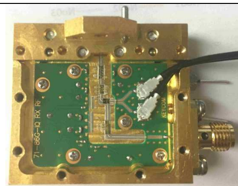
Rx Module
