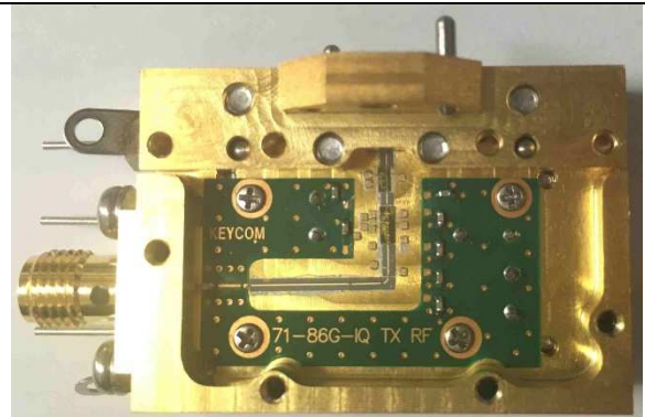
Tx Module
