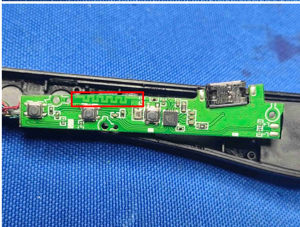
Antenna
