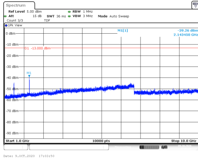
Band12-3MHz-QPSK-23165-15RB#0-Range2:1000~10000MHz--39.26-PASS
