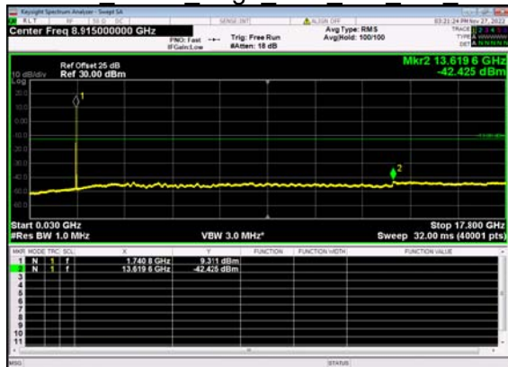
N66(10M)_DFT-s- OFDM BPSK Edge 1RB Left Mid CH
