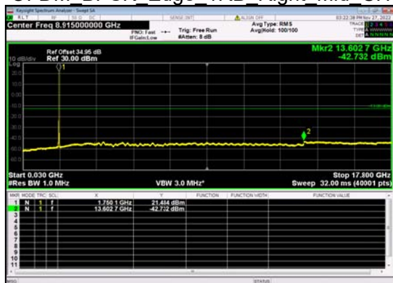
N66(10M)_DFT-s- OFDM BPSK Edge 1RB Right Mid CH
