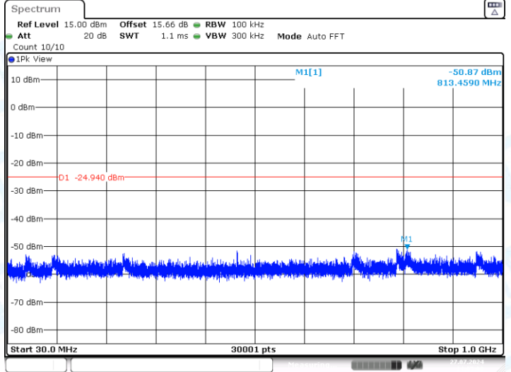
11G-Ant1-2412-30~1000-PASS
