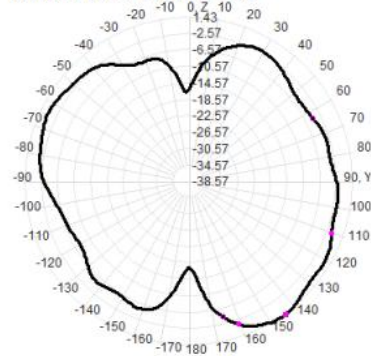
2400.0MHz Total(E2-YZ), Max= 1.43dBi
