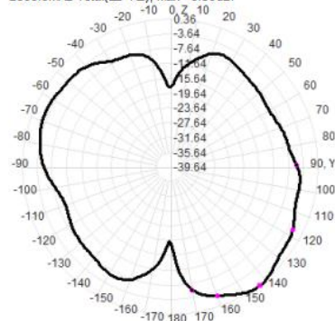
2500.0MHz Total(E2-YZ), Max= 0.36dBi
