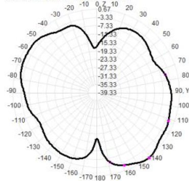
2450.0MHz Total(E2-YZ), Max= 0.67dBi
