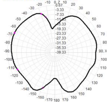
2450.0MHz Total(E1-XZ), Max=-1.63dBi
