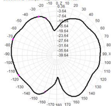
2500.0MHz Total(E1-XZ), Max=-1.81dBi
