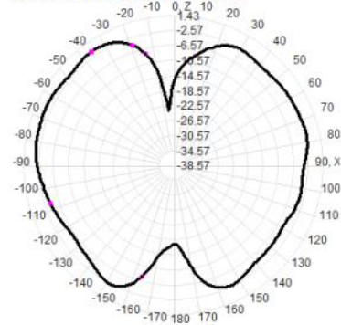
2400.0MHz Total(E1-XZ), Max=-1.12dBi
