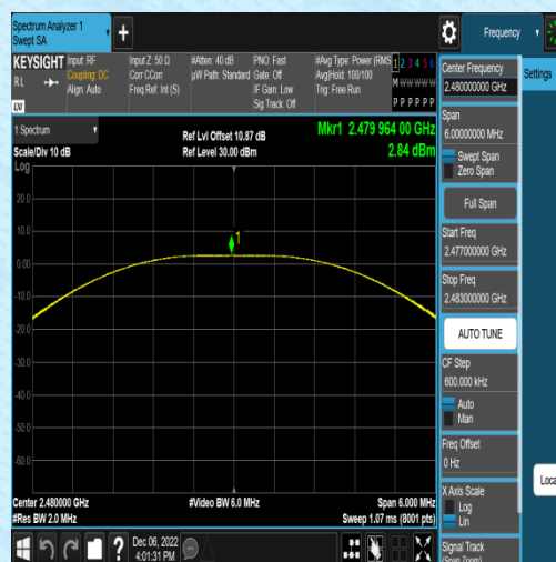
BLE_2M-Ant1-2480
