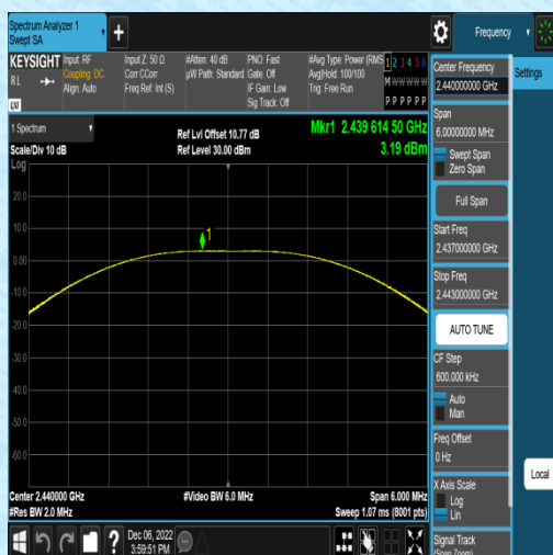
BLE_2M-Ant1-2440
