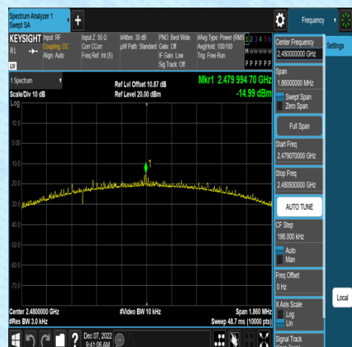
BLE_2M-Ant1-2480
