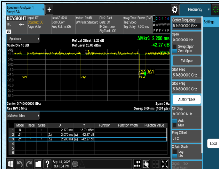
NTNV-11A-Ant1-5745
