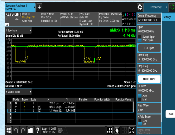
NTNV-11N40MIMO-Ant1-5190
