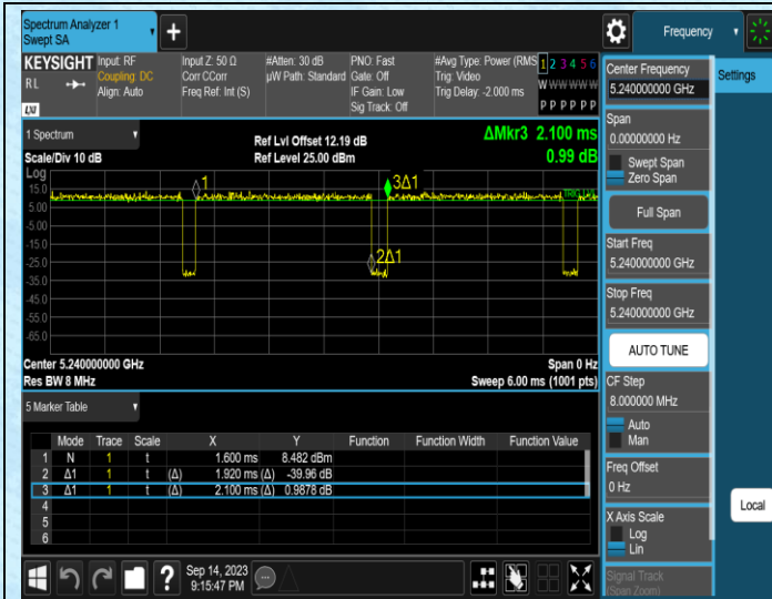
NTNV-11N20MIMO-Ant1-5240
