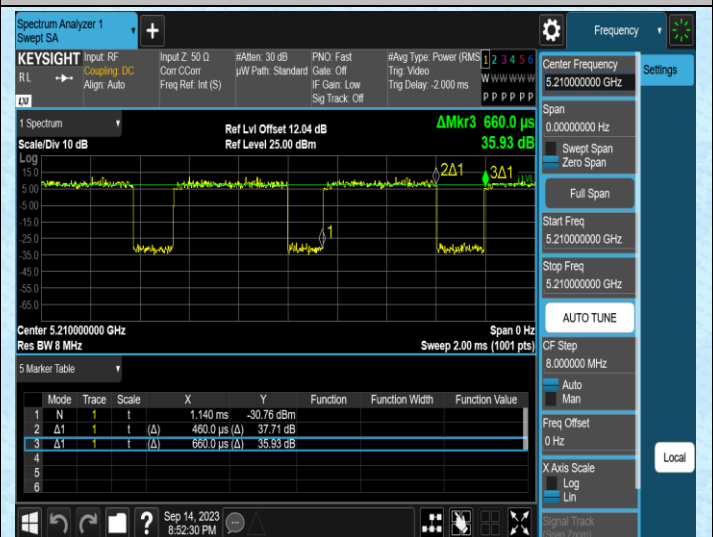
NTNV-11AC80SISO-Ant2-5210
