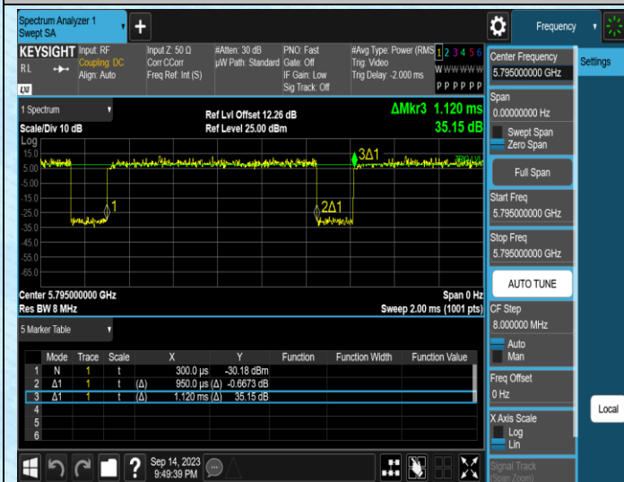
NTNV-11N40MIMO-Ant1-5795
