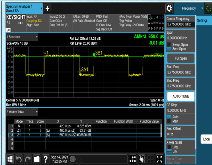
NTNV-11AC80SISO-Ant1-5775
