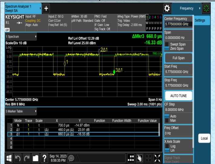
NTNV-11AC80SISO-Ant2-5775
