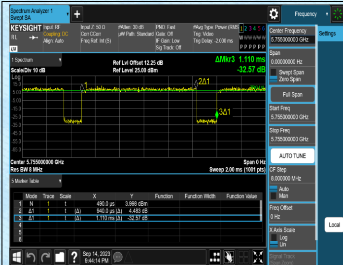
NTNV-11N40MIMO-Ant1-5755
