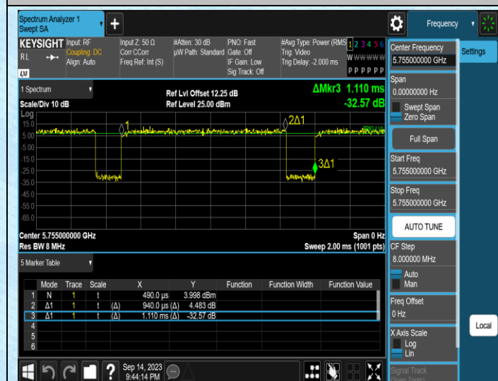
NTNV-11N40MIMO-Ant1-5755
