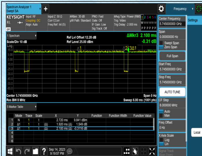
NTNV-11N20MIMO-Ant1-5745
