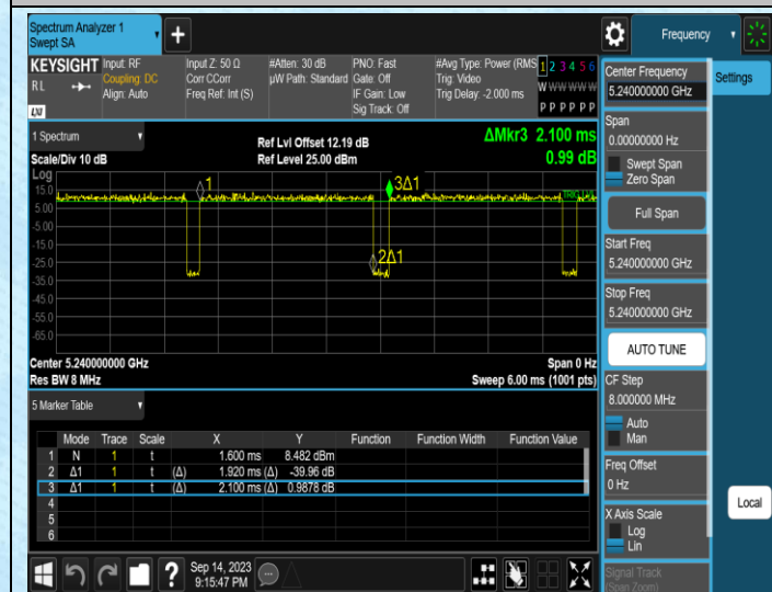
NTNV-11N20MIMO-Ant1-5240
