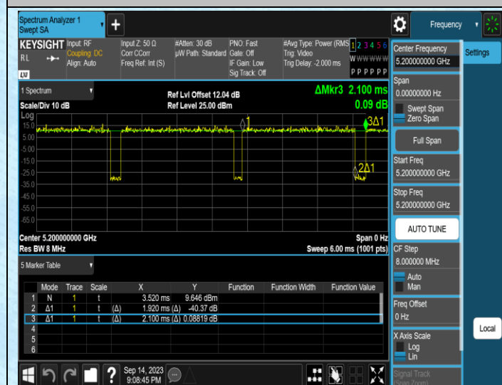
NTNV-11N20MIMO-Ant1-5200
