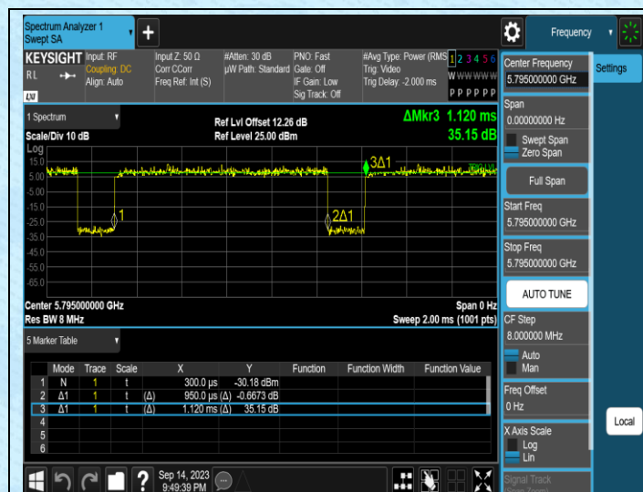
NTNV-11N40MIMO-Ant1-5795
