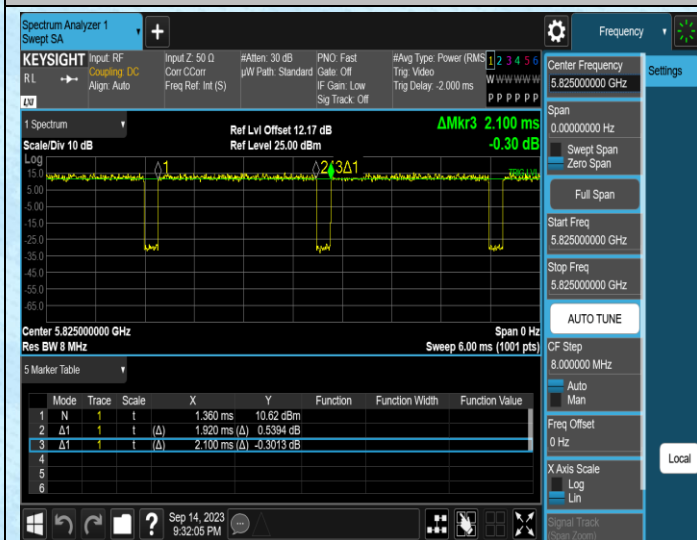
NTNV-11N20MIMO-Ant1-5825
