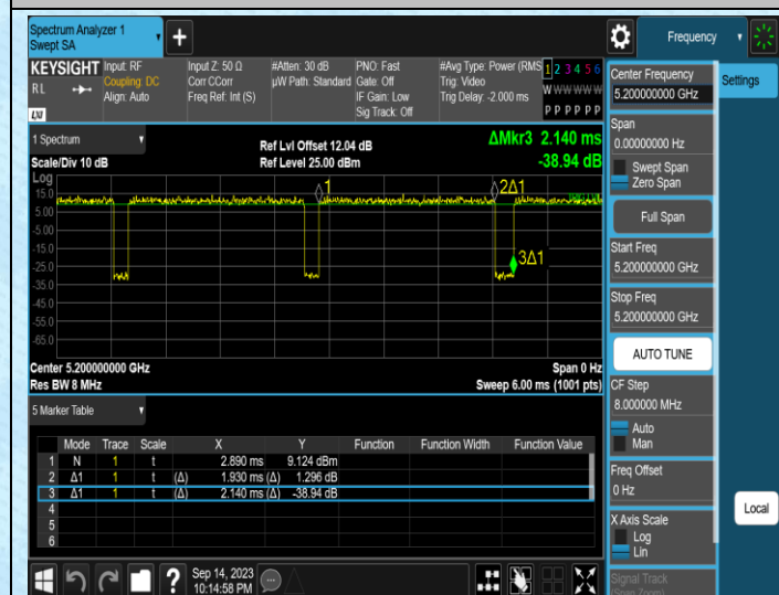
NTNV-11AC20MIMO-Ant1-5200
