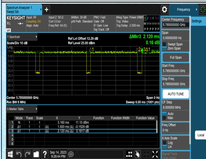
NTNV-11N20MIMO-Ant1-5785
