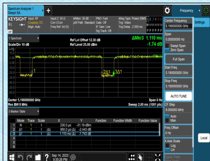
NTNV-11N40MIMO-Ant1-5190
