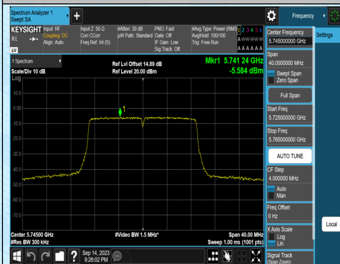
11N20MIMO-Ant1-5745
