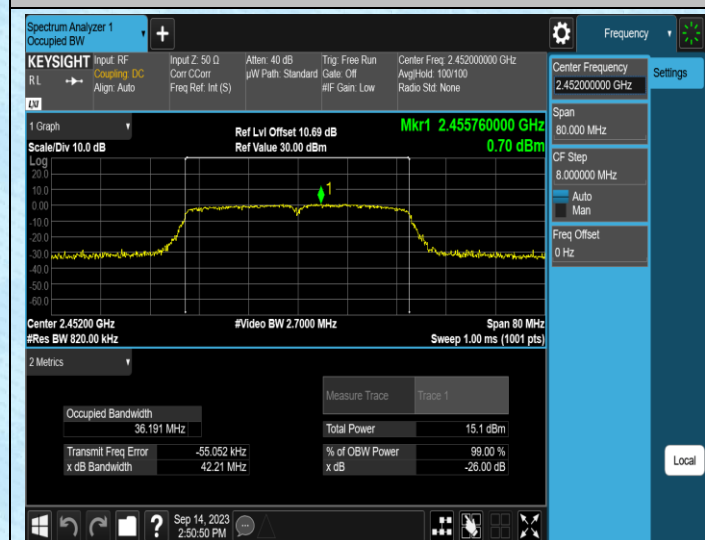
11N40MIMO-Ant1-2452
