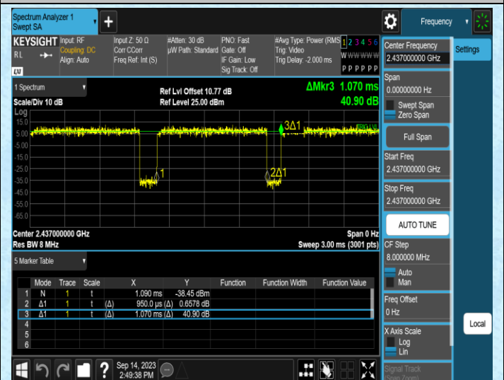
NTNV-11N40MIMO-Ant2-2437
