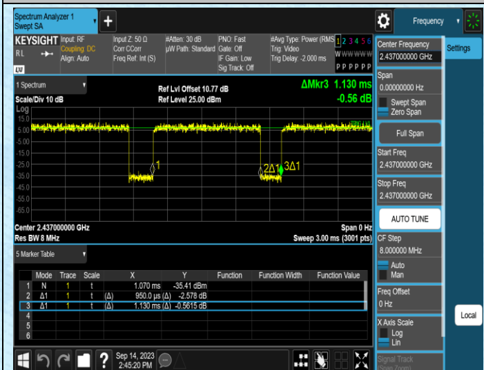
NTNV-11N40MIMO-Ant1-2437
