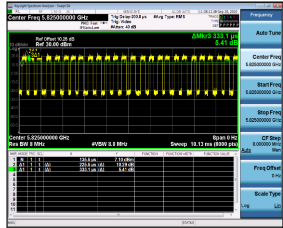
802.11ac(HT40)
