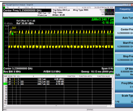
802.11ac(HT40)
