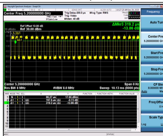
802.11ac(HT20)
