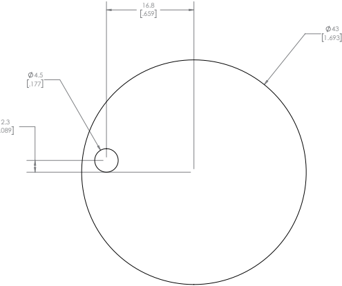
尺寸刀模示意
