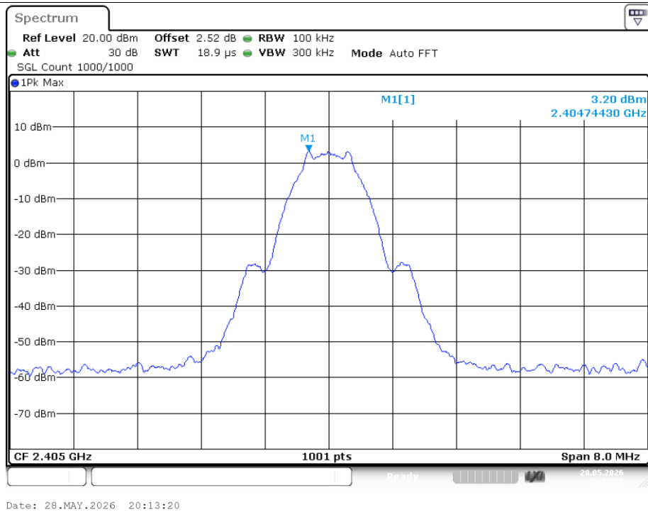
Band Edge NVNT 2.4G 2405MHz Ant1 Ref
