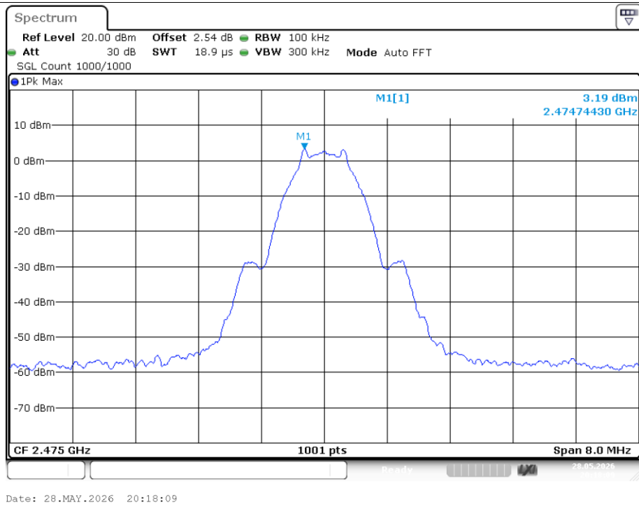
Band Edge NVNT 2.4G 2475MHz Ant1 Ref
