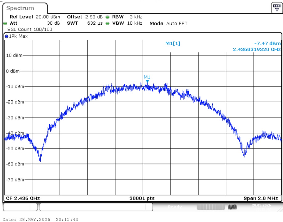
PSD NVNT 2.4G 2436MHz Ant1
