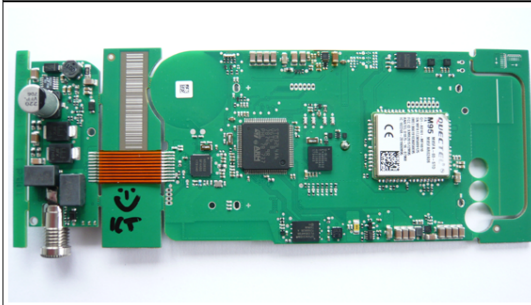
PCB Top
