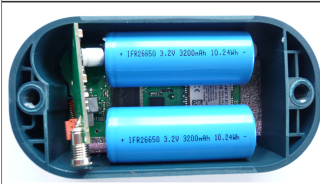
EUT Internal
