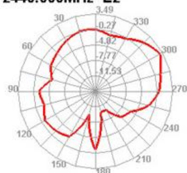
2440.000MHz E2
