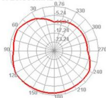
5720.000MHz H
