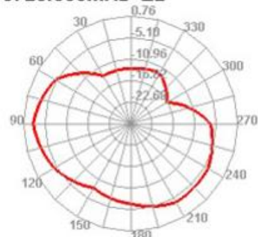
5720.000MHz E2
