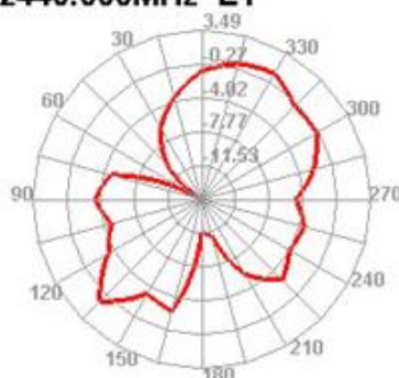
2440.000MHz E1
