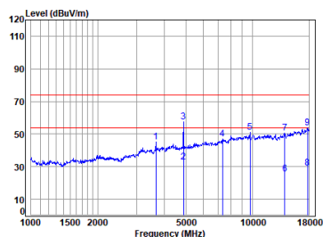
BT_DH5_TX_CH_39_Horizontal
