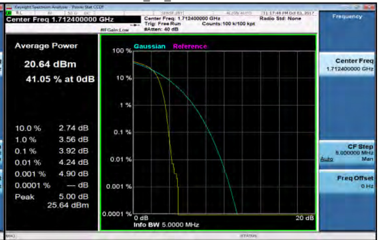
HSUPA_B4_LowCH1312-1712.4
