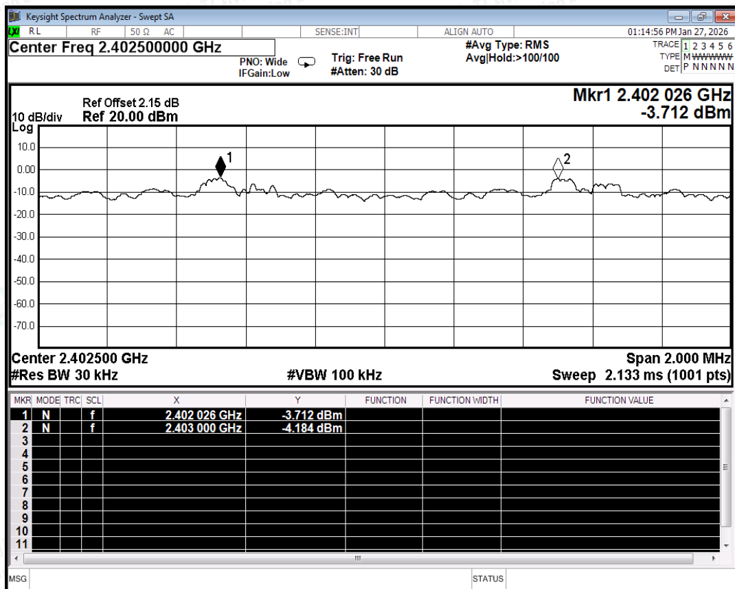
CFS NVNT 2-DH5 2402MHz Ant0
