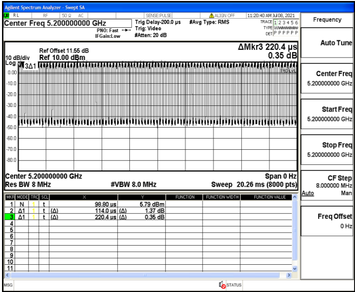
11AX20MIMO_Ant2_5200
